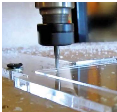
Мал. 197. Фрезерування пластику
