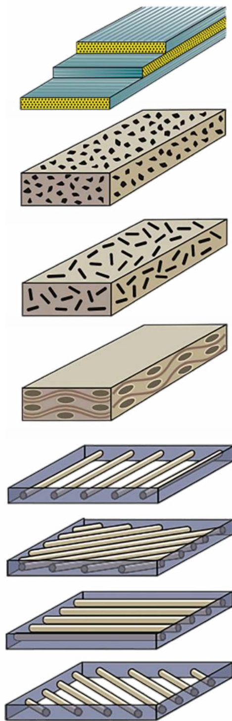
Мал. 155. Різні за формою наповнювачі та їхня орієнтація
