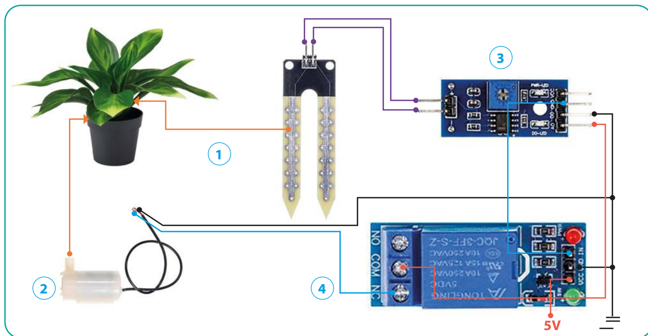
Мал. 217. Принципова схема підключення автоматичного поливу: 1) щуп датчика вологості; 2) мініпомпа; 3) датчик вологості; 4) реле
