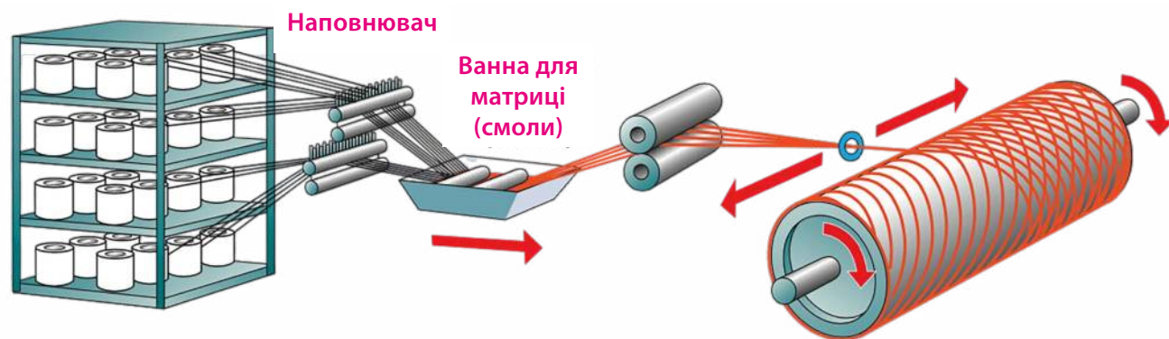
Мал. 156. Схема виготовлення корпусів ракетних двигунів
