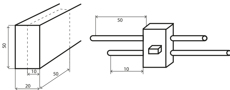
Мал. 83. Розмічання рейсмусом
