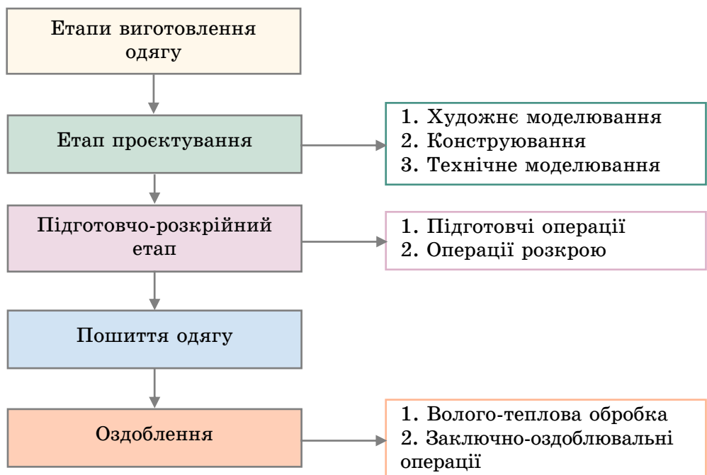
Рис. 4.7. Процес виготовлення одягу
