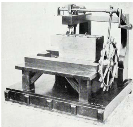
Швейні машини Томаса Сейнта (1790 р.) та Еліаса Гоу (1845 р.)
