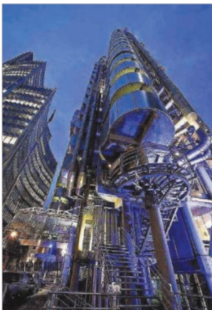
Будівля страхової компанії «Ллойдс» у Лондоні, Велика Британія. Арх. Р. Роджерс та ін., 1978–1986 рр.
