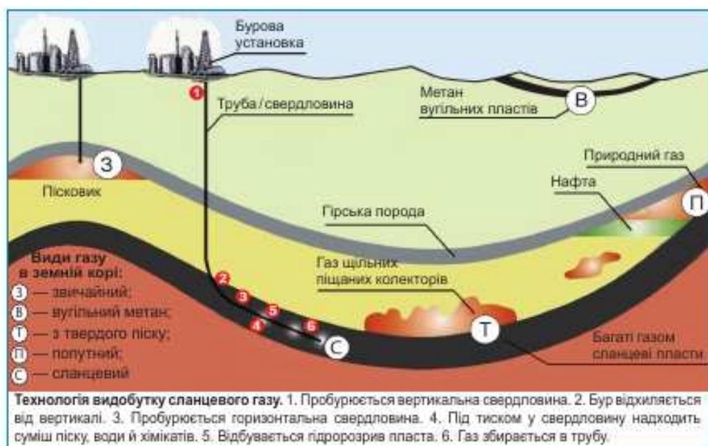
Мал. 83. Схема залягання та видобутку сланцевого газу
