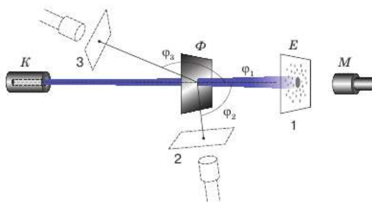
Мал. 30.2. Схема досліді Резерфорда
