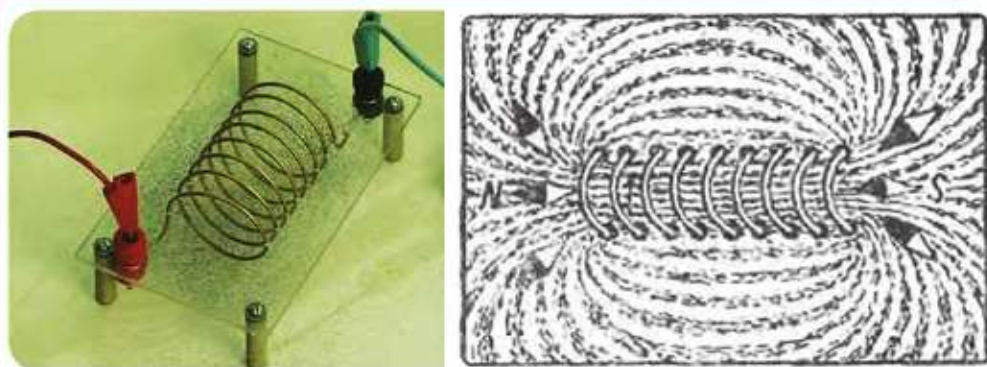
Мал. 17.2. Дослідження магнітного поля котушки зі струмом:
