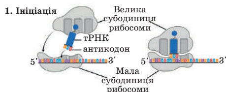
Мал. 28.8. Ініціація
