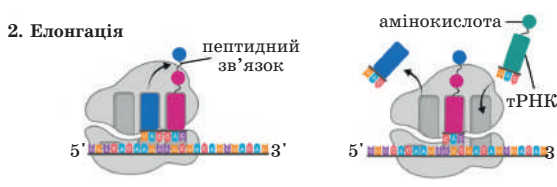
Мал. 28.9. Елонгація
