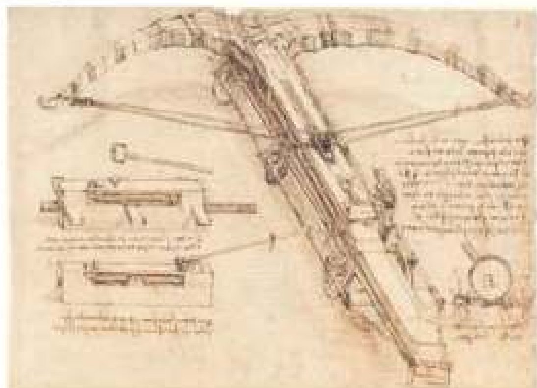
Креслення Леонардо да Вінчі. Близько 1500 р.
