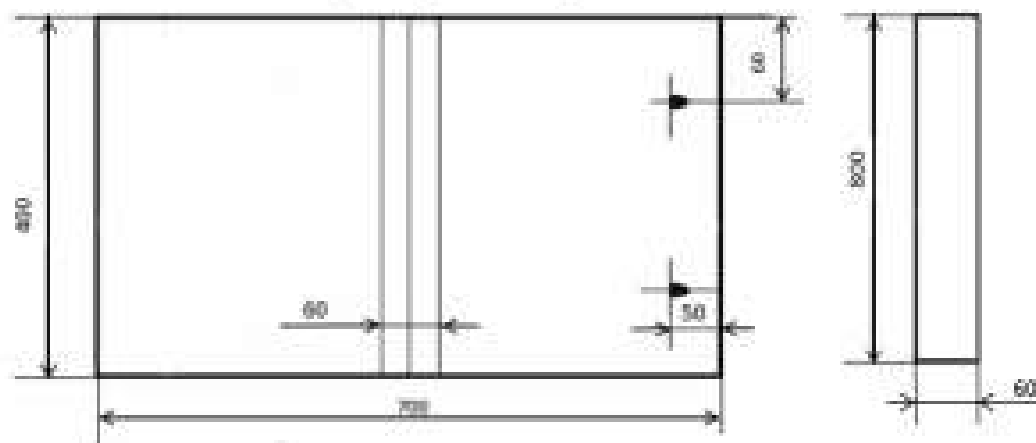
Креслення деталей торбини
