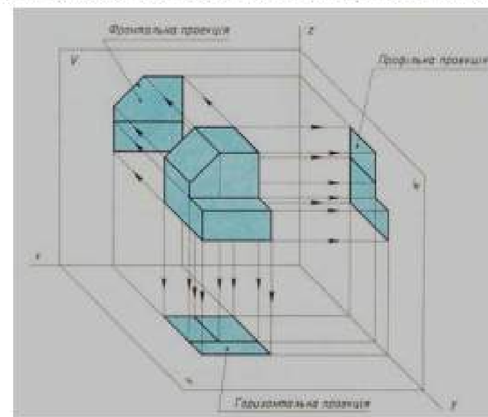
Рис. 1.14. Проекція предмета на три площини
