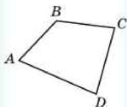
Чотирикутник ABCD
