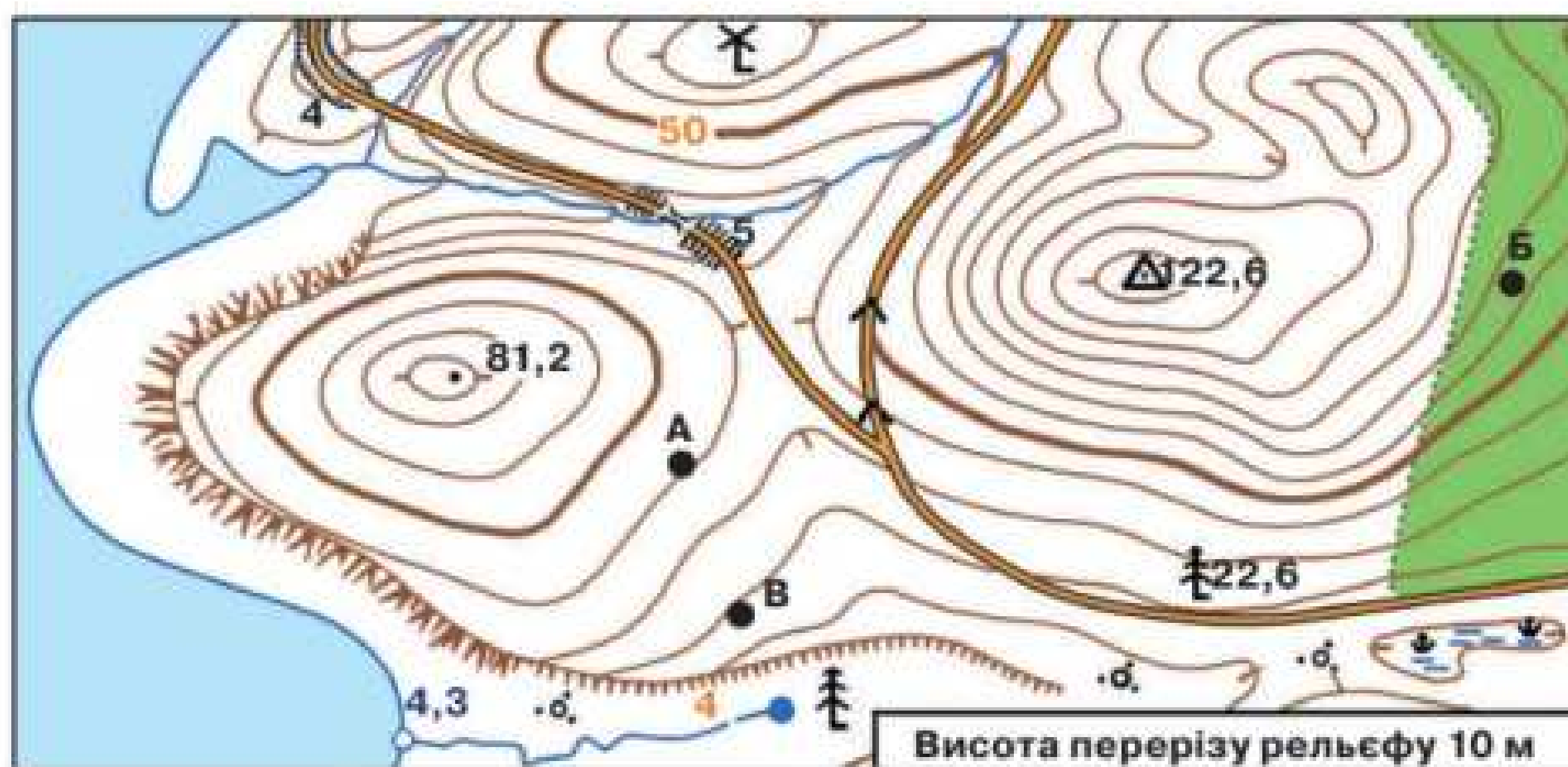
Мал. 7.4. Зображення рельєфу на топографічній карті масштабу 1: 5000
