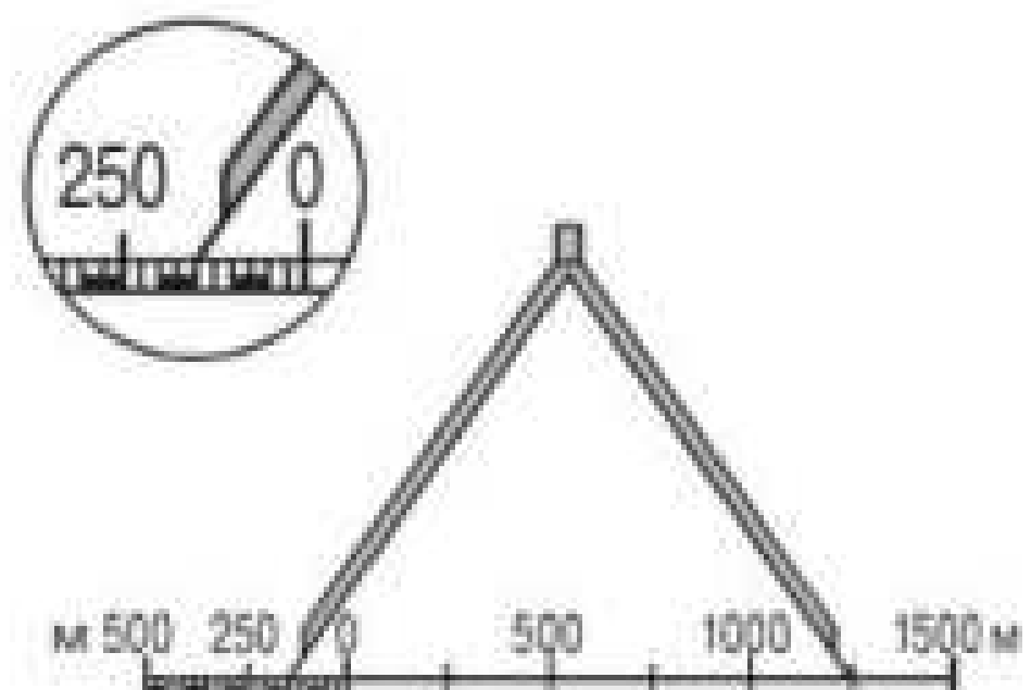
Мал. 8.1. Вимірювання відстаней на топографічній карті за допомогою циркуля-вимірювача
