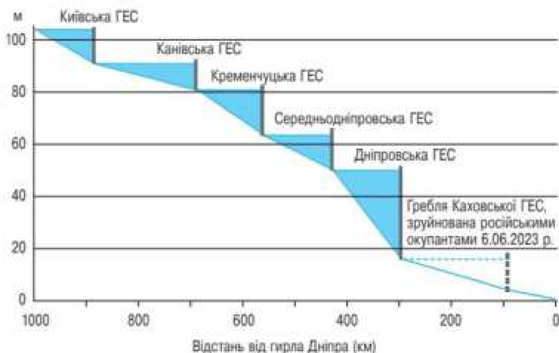
Мал. 38.2. Зарегулювання річки Дніпро каскадом водосховищ
