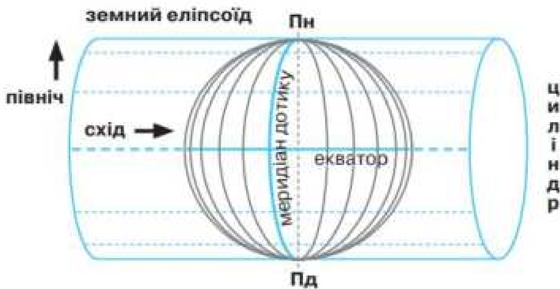
Мал. 7.1. Побудова 6 а колон у поперечно-циліндричній рівнокутній проекції Гаусса-Крюгера
