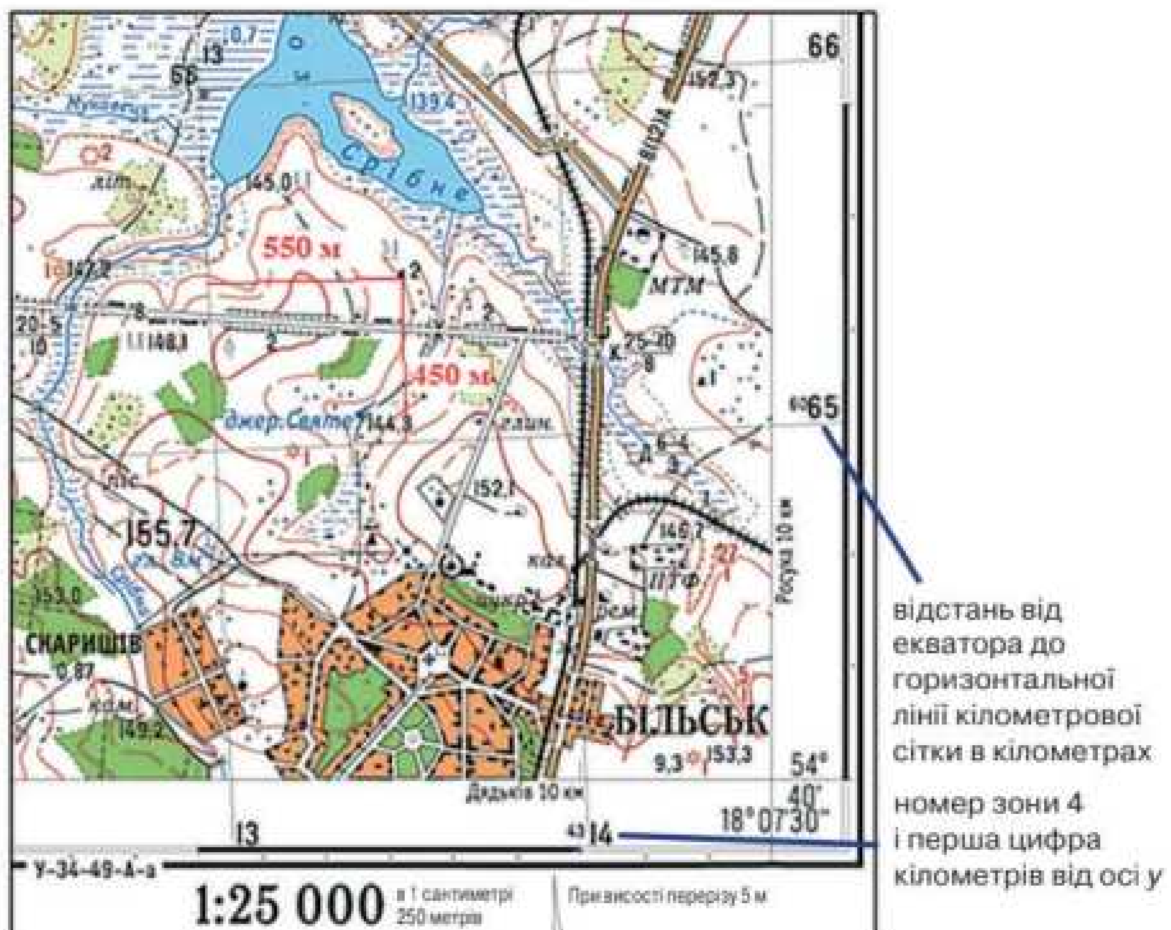
Мал. 8.4. Визначення прямокутних координат точки на топографічній карті
