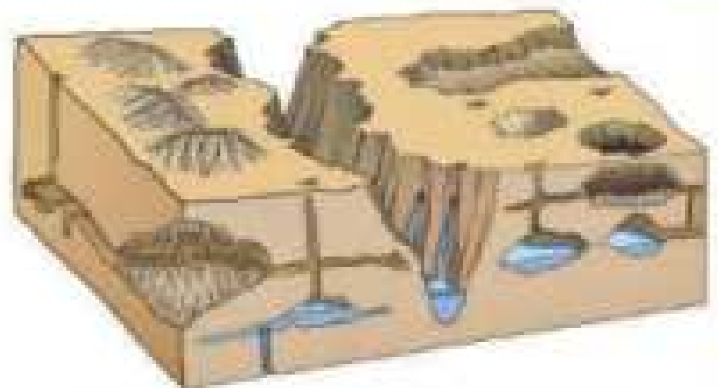
Процеси рельєфоутворення. Схематичний малюнок
