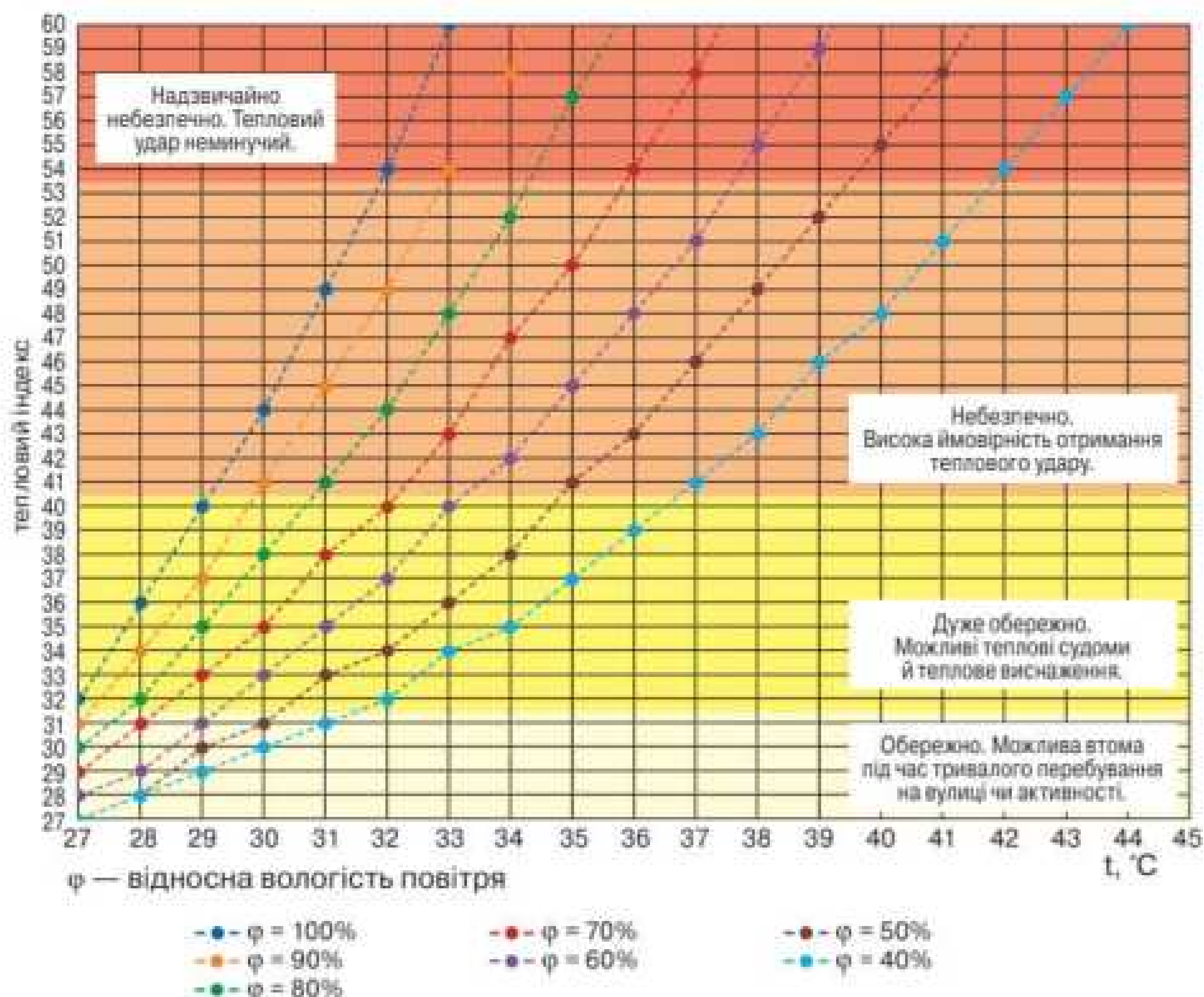
Мал. 18.3. Графіки, за допомогою яких визначають тепловий індекс
