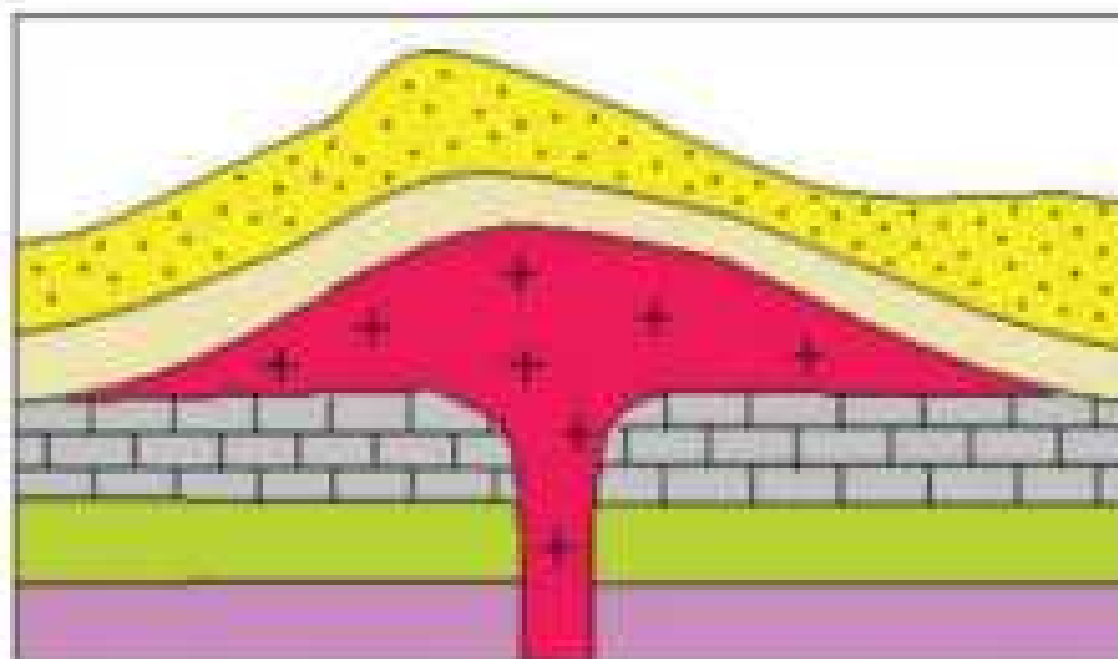
Мал. 13.2. Схема утворення лаколіту
