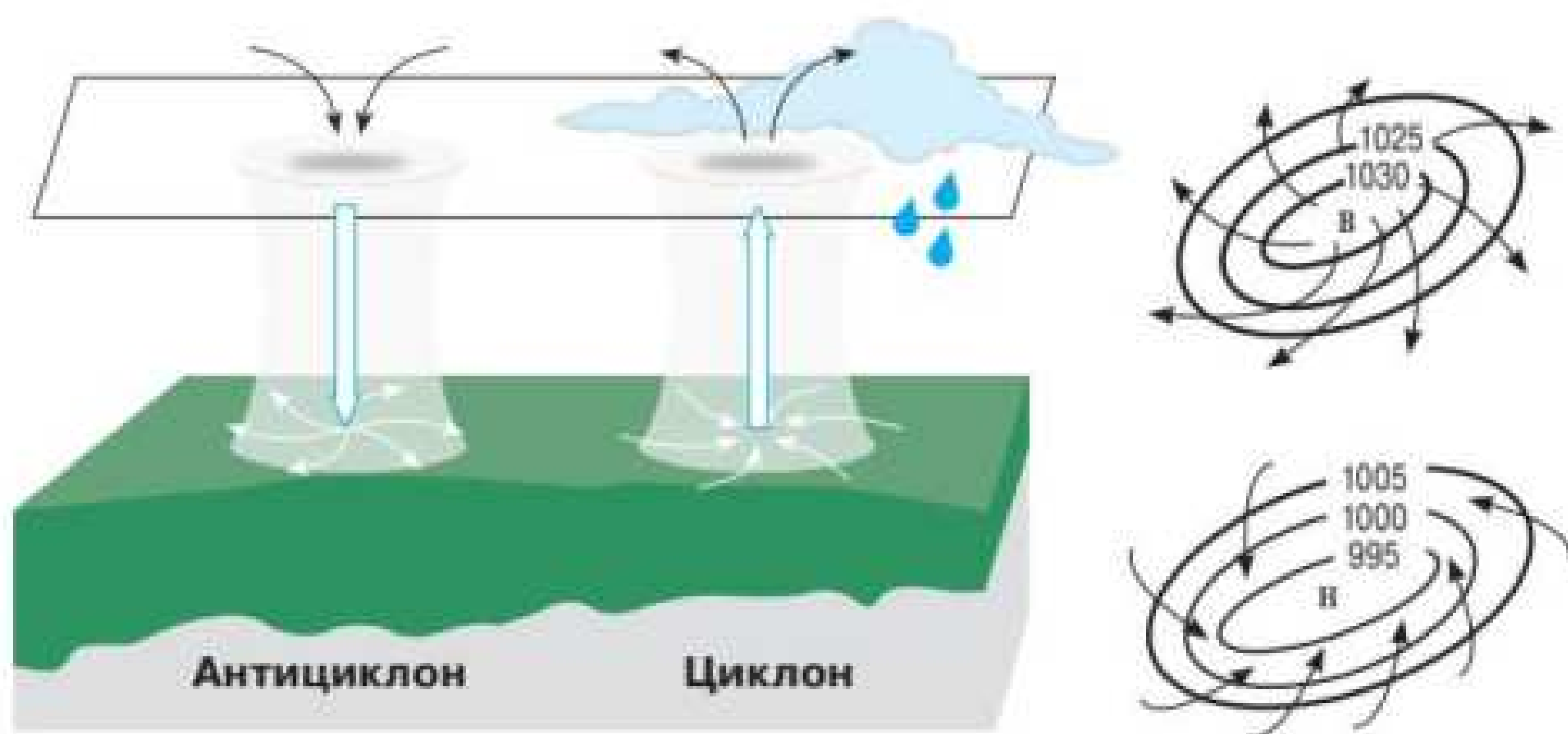
Мал. 15.6. Схеми антициклону й циклону в Північній півкулі та їх зображення на синоптичних картах
