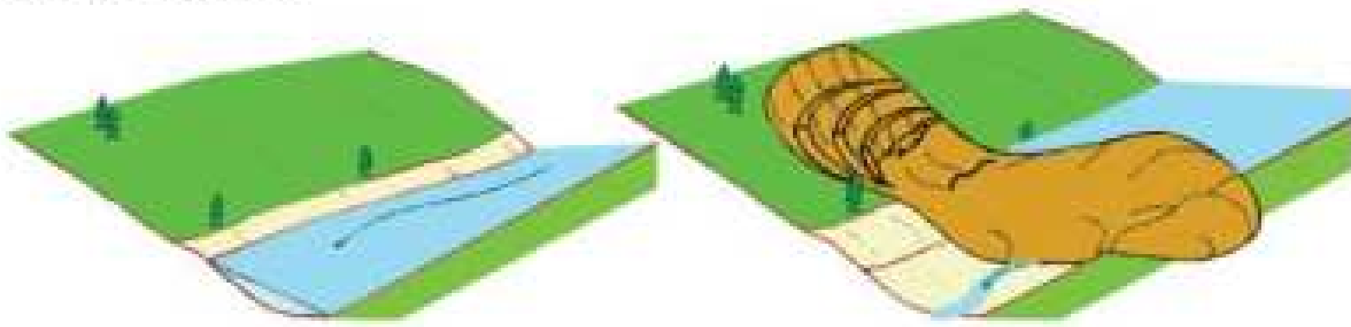
Мал. 20.4. Схема утворення загатного озера
