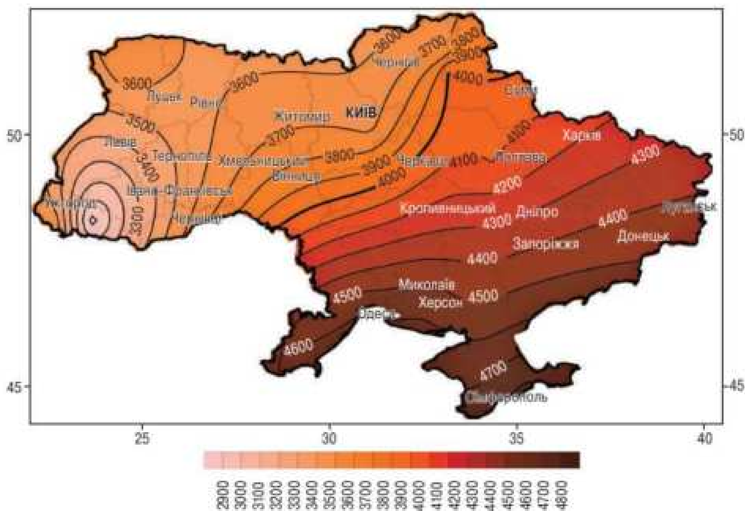
Мал. 15.2. Середньорічна кількість сумарної сонячної радіації (МДж/м 2 ) у 2001–2010 рр.
