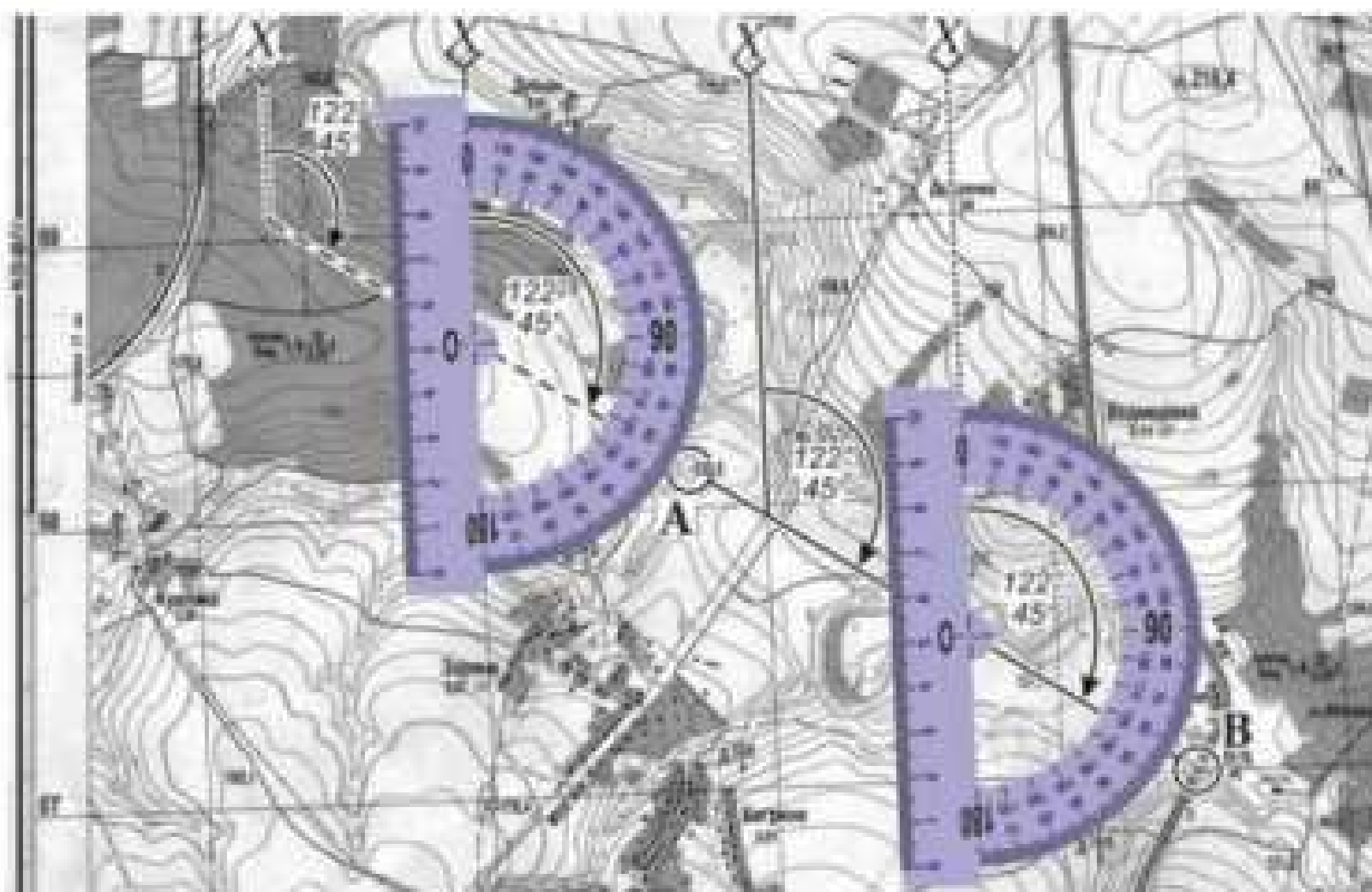
Мал. 39. Визначення за топографічною картою дирекційного кута
