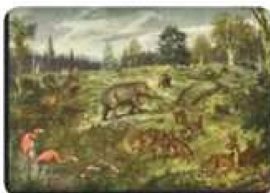
Мал. 76. Розвиток життя на Землі в періоди Кайнозою
