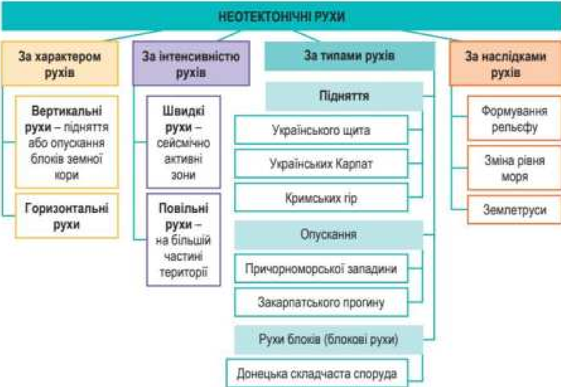
Мал. 81. Неотектонічні рухи на території України
