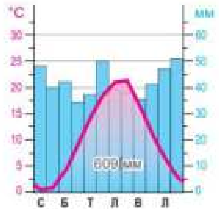
Мал. 109. Кліматодіаграма м. Ялта
