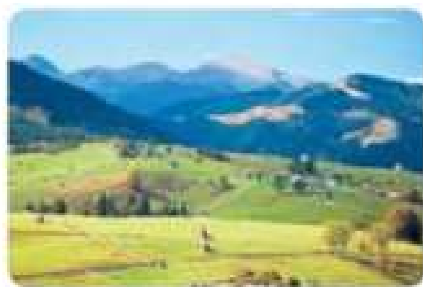
Мал. 174. Полонини Карпат
