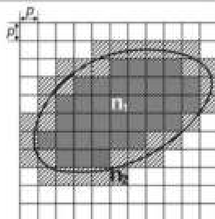
Мал. 46. Квадратна палетка
