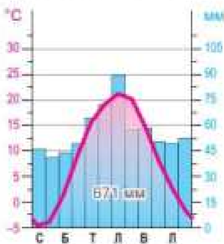
Мал. 160. Кліматодіаграма м. Чернівці
