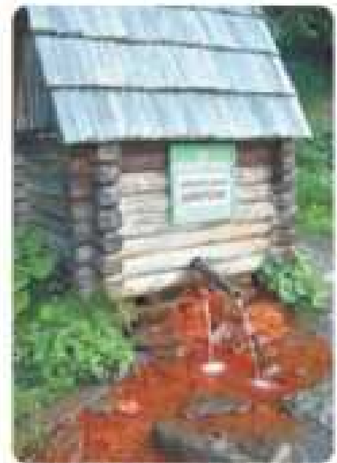
Мал. 136. Джерело природної газованої води в селі Калечин
