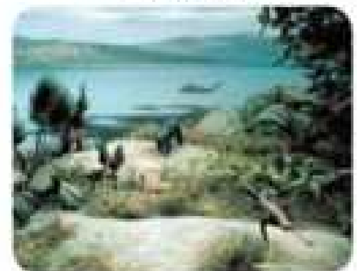
Мал. 75. Розвиток життя на Землі в періоди Мезозою
