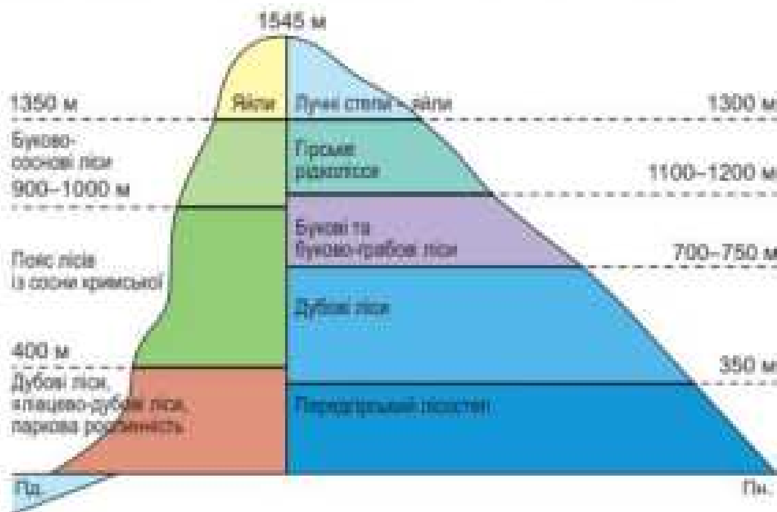
Мал. 176. Вертикальна поясність Кримських гір
