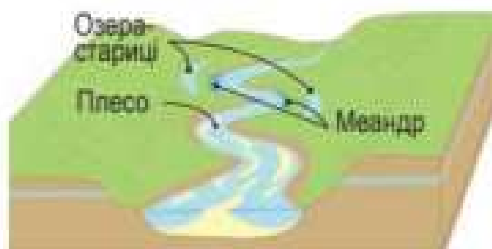
Мал. 120. Утворення меандрів на річках
