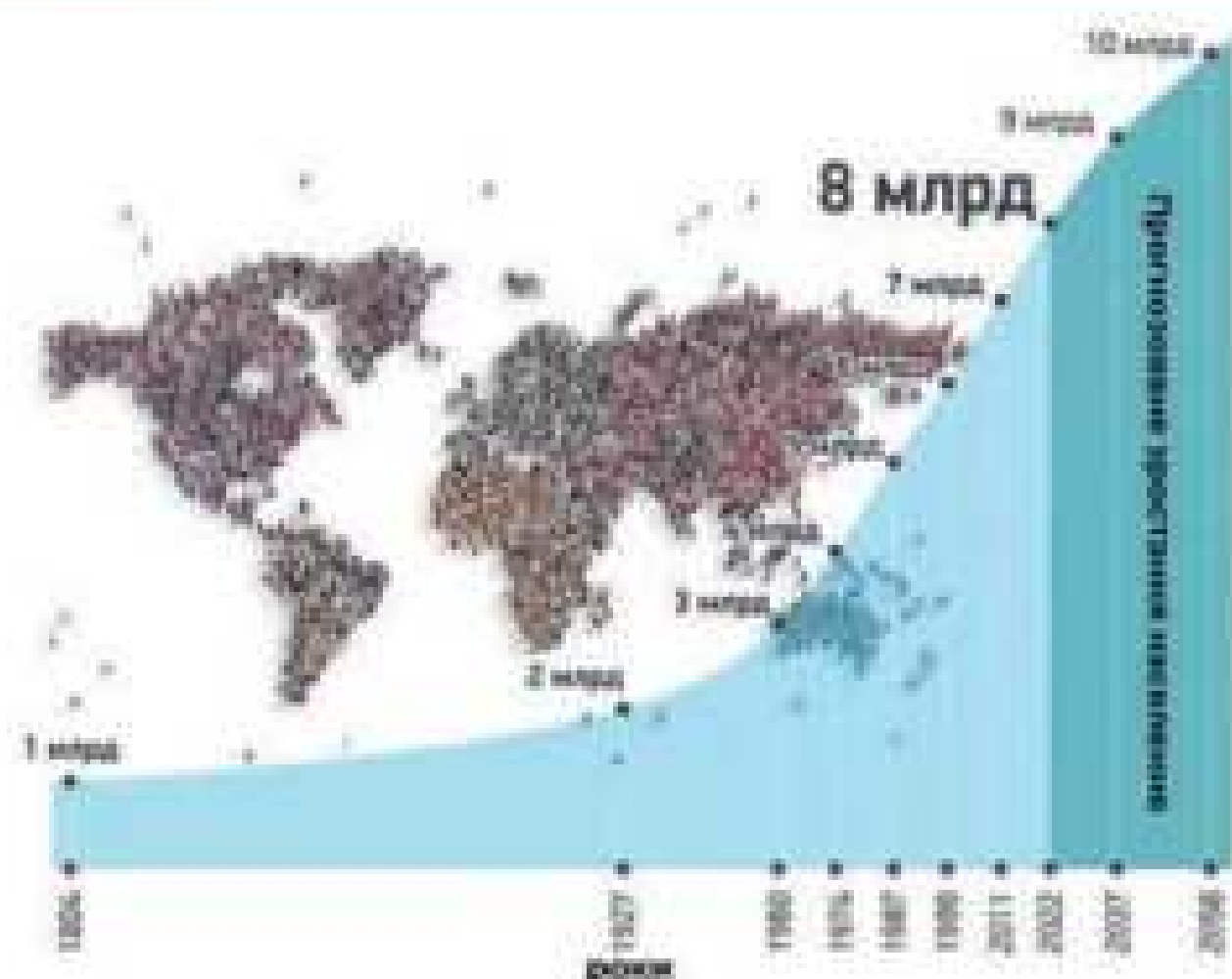
Мал. 196. Динаміка чисельності населення на Землі
