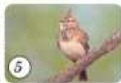
Мал. 171. Типові рослини і тварини степової зони: 1 – ковила; 2 – тонконіг, 3 – ховрах, 4 – гадюка степова, 5 – жайворонок
