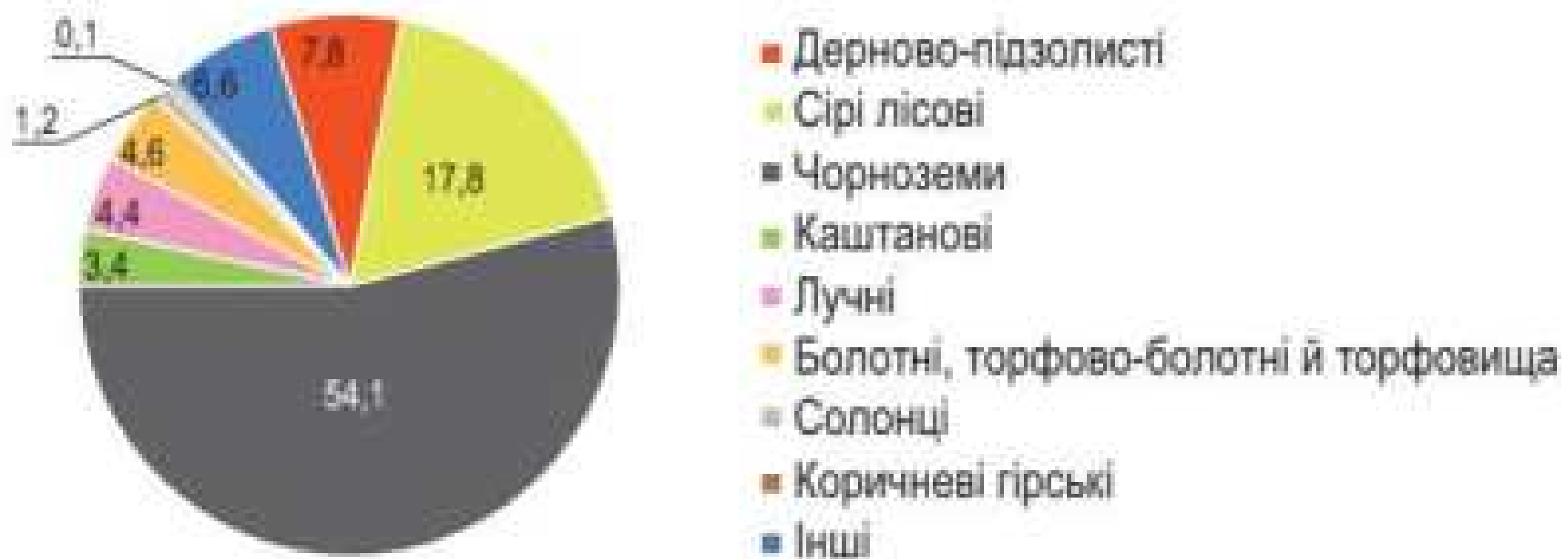
Мал. 145. Площі основних типів ґрунтів України, %
