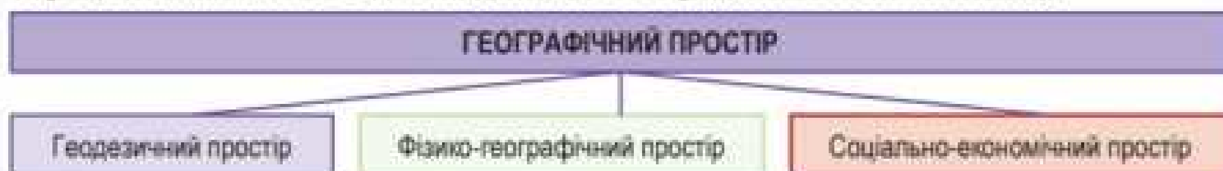
Мал. 49. Складники географічного простору
