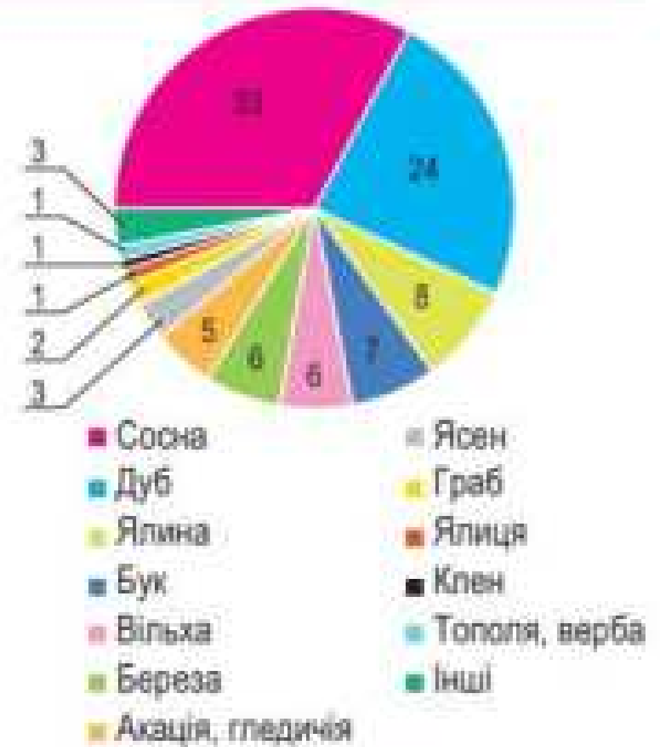
Мал. 150. Розподіл площі лісів України за переважаючими деревними породами, %
