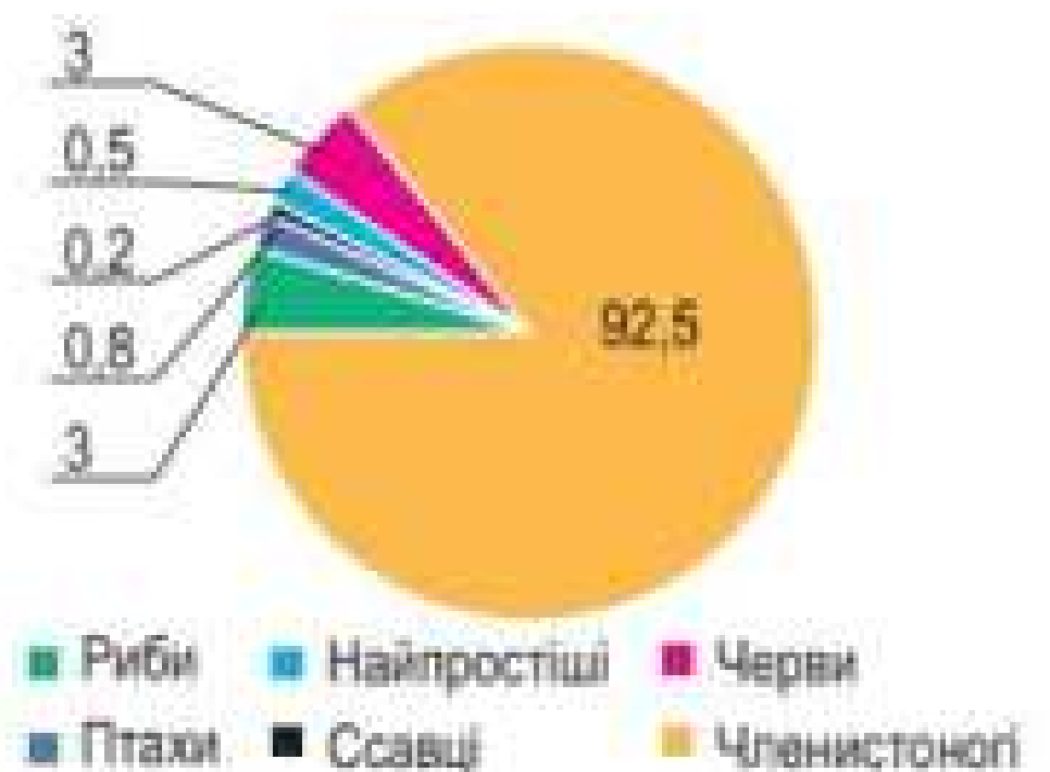
Мал. 154. Структура фауни території України, %
