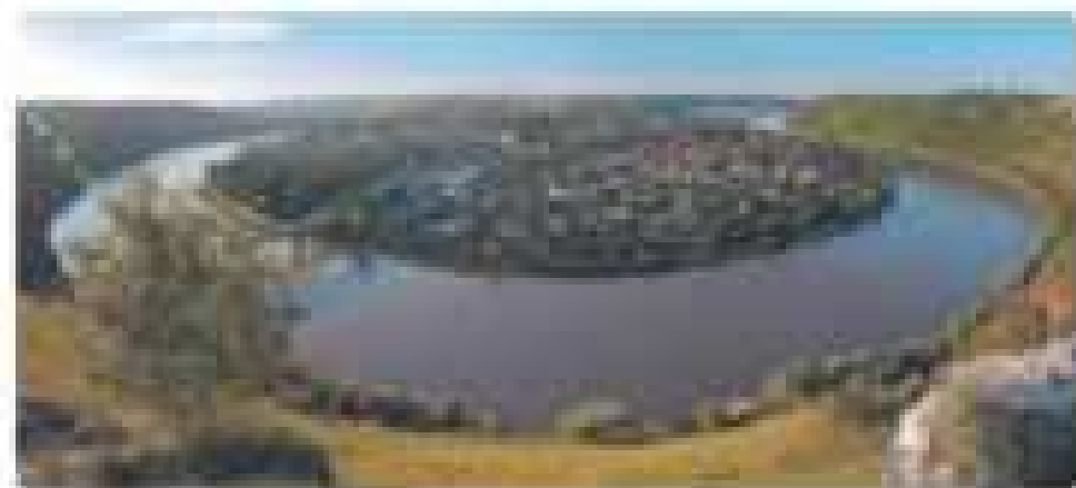
Мал. 121. Меандр на річці Дністер біля селища Заліщики
