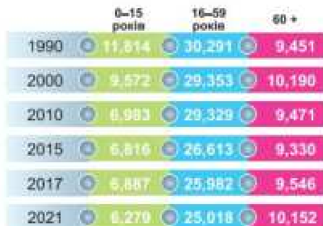
Мал. 214. Віковий розподіл населення, млн осіб
