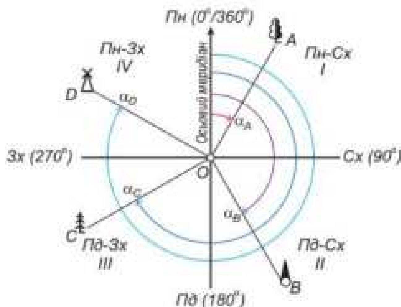
Мал. 38. Дирекційні кути напрямків
