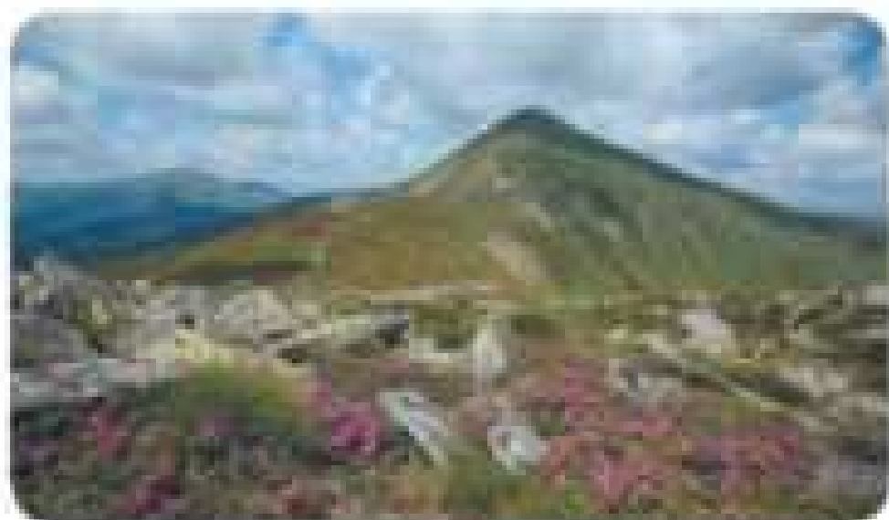
Мал. 172. Масив Чорногора з вершиною г. Говерла
