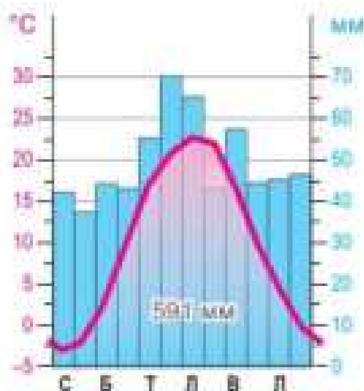
Мал. 166. Кліматодіаграма м. Черкаси
