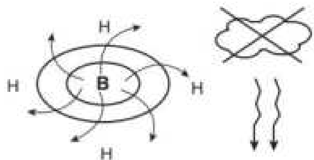
Мал. 100. Формування антициклонів у Північній півкулі
