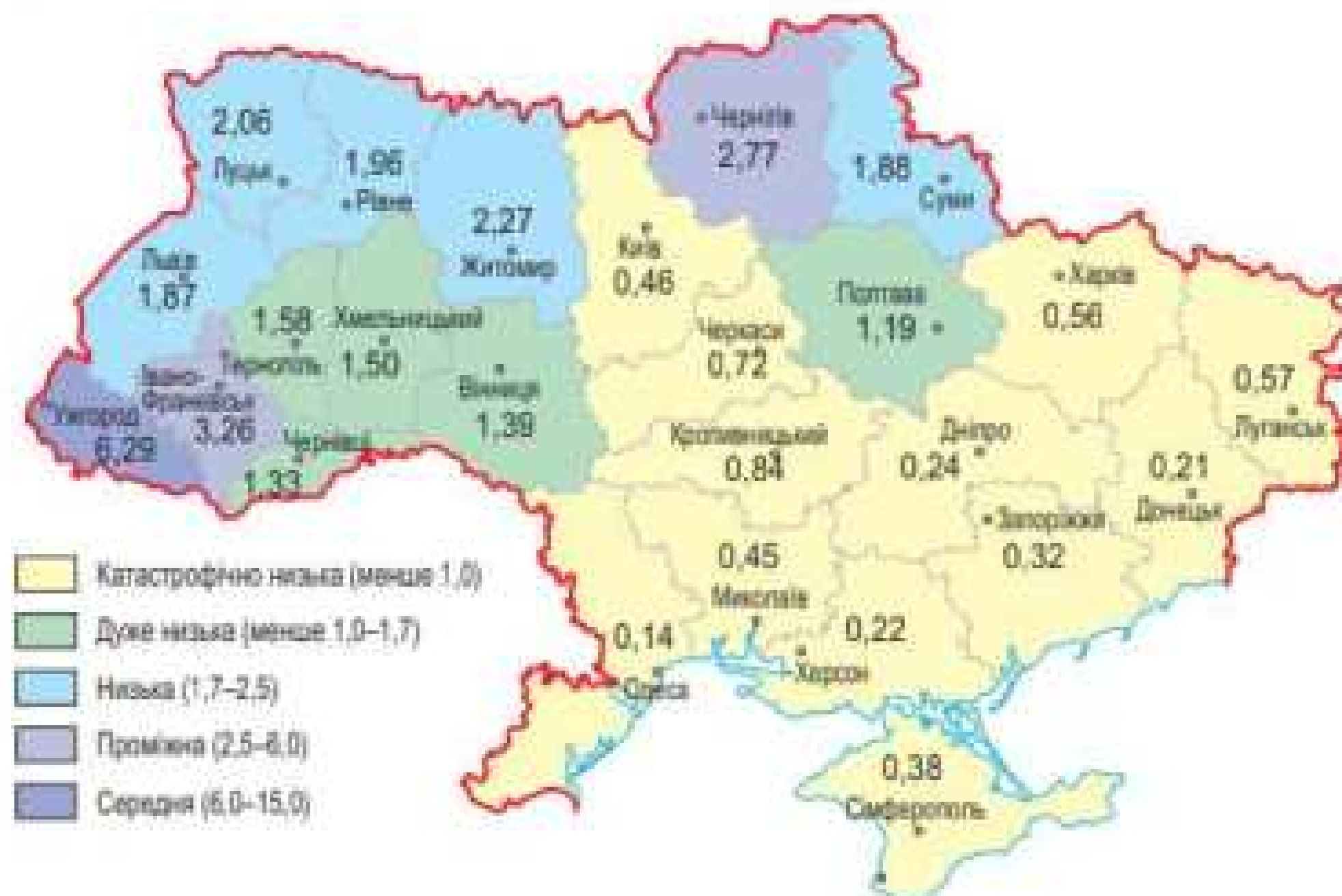
Мал. 137. Забезпеченість областей України водними ресурсами (тис. м³ на рік на одну людину)
