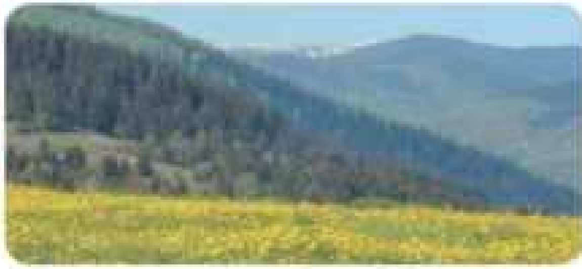
Мал. 151. Карпатські луки
