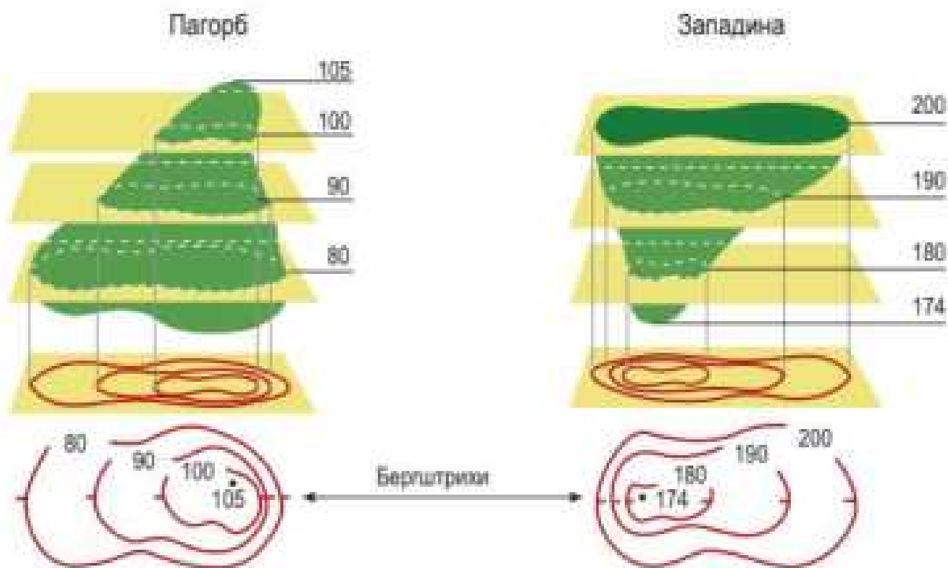
Мал. 48. Застосування бергштрихів на карті
