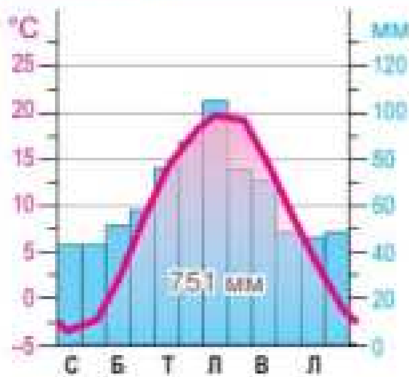
Мал. 163. Кліматодіаграма м. Тернопіль
