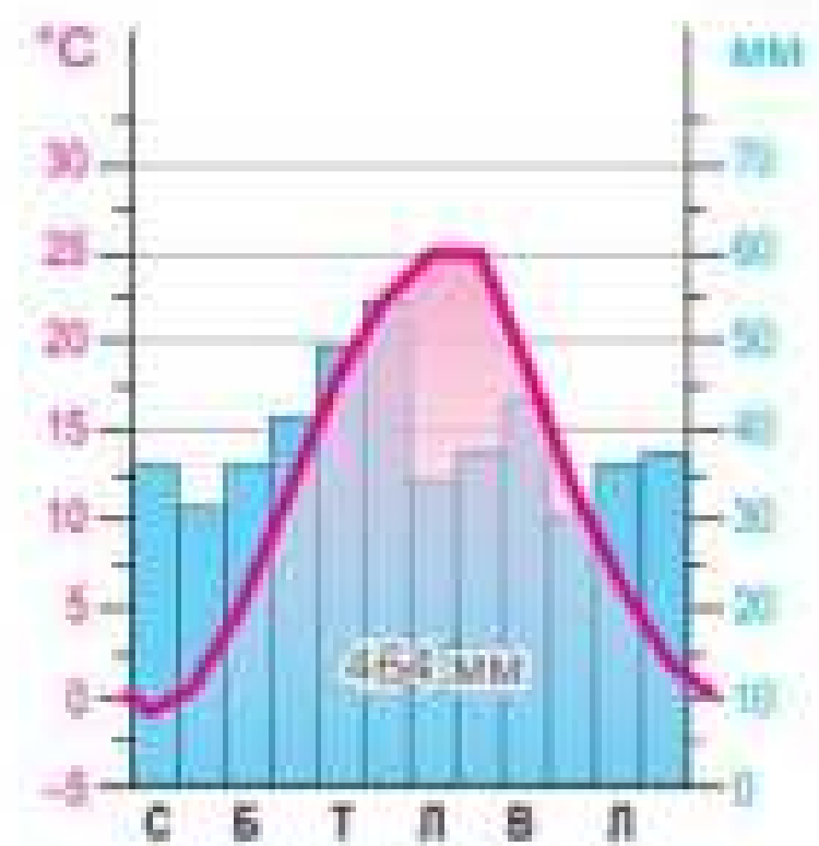
Мал. 170. Кліматодіаграма м. Херсон
