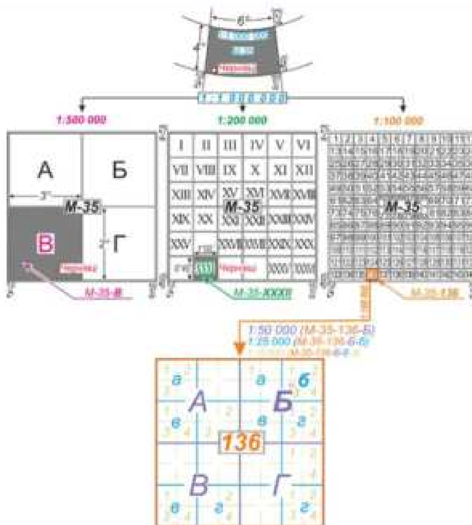
Мал. 30. Розграфлення топографічних карт масштабного ряду 1:1 000 000 – 1:10 000
