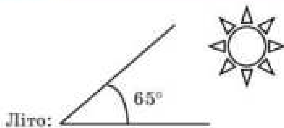
Мал. 95. Висота Сонця над горизонтом у день літнього сонцестояння в географічному центрі України ( 48^{\circ}32' пн. ш.)
