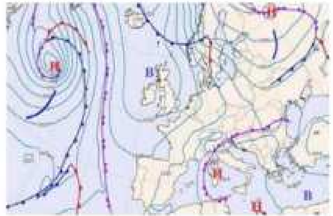
Мал. 114. Синоптична карта Європи (на 03.03.2023, 12 год)
