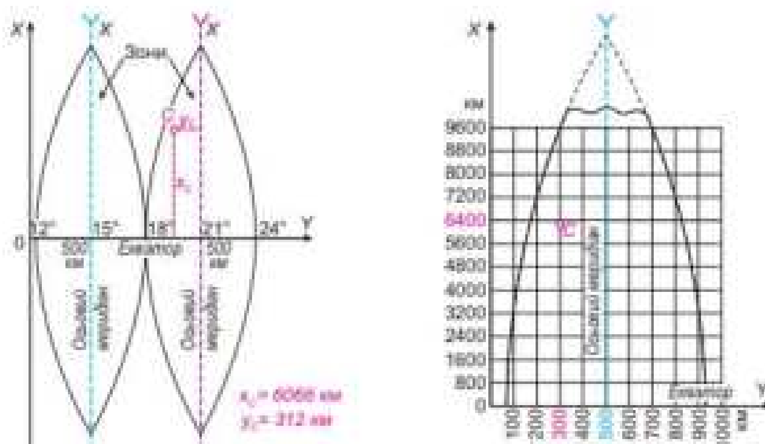
Мал. 34. Зональна система плоских прямокутних координат
