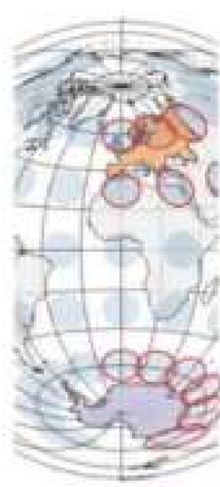
Мал. 24. Рівнопроміжна проєкція
