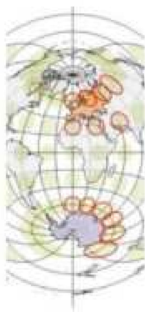
Мал. 23. Рівновелика проєкція
