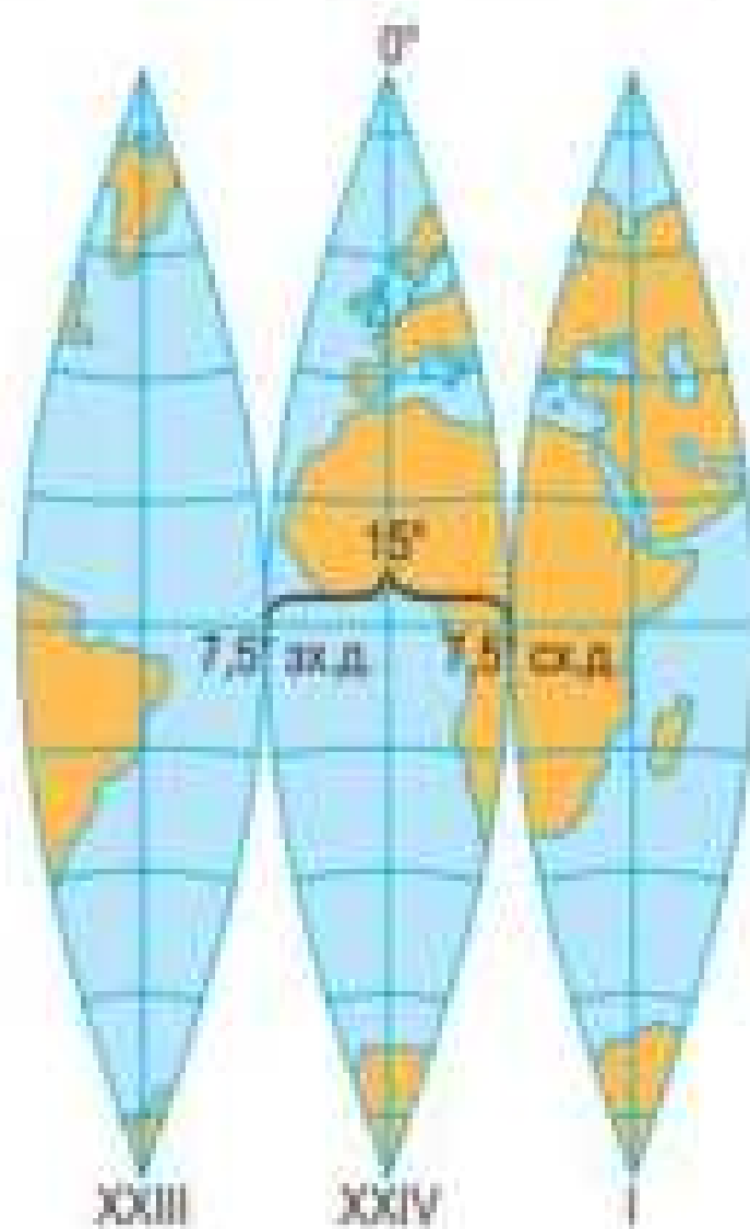
Мал. 63. Середній меридіан
