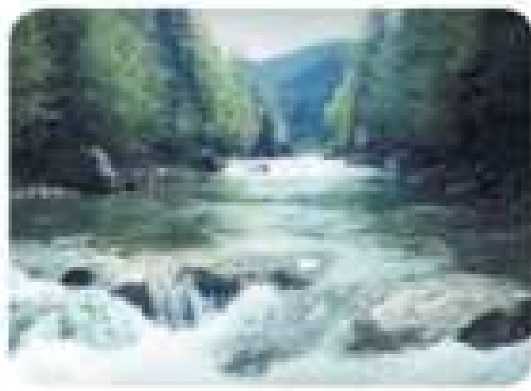
Мал. 123. Пороги на р. Прут
