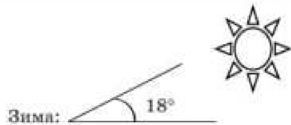
Мал. 96. Висота Сонця над горизонтом у день зимового сонцестояння в географічному центрі України ( 48^{\circ}32' пн. ш.)
