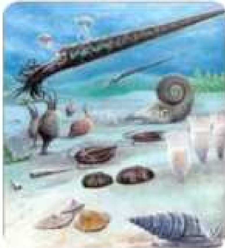
Ордовик
