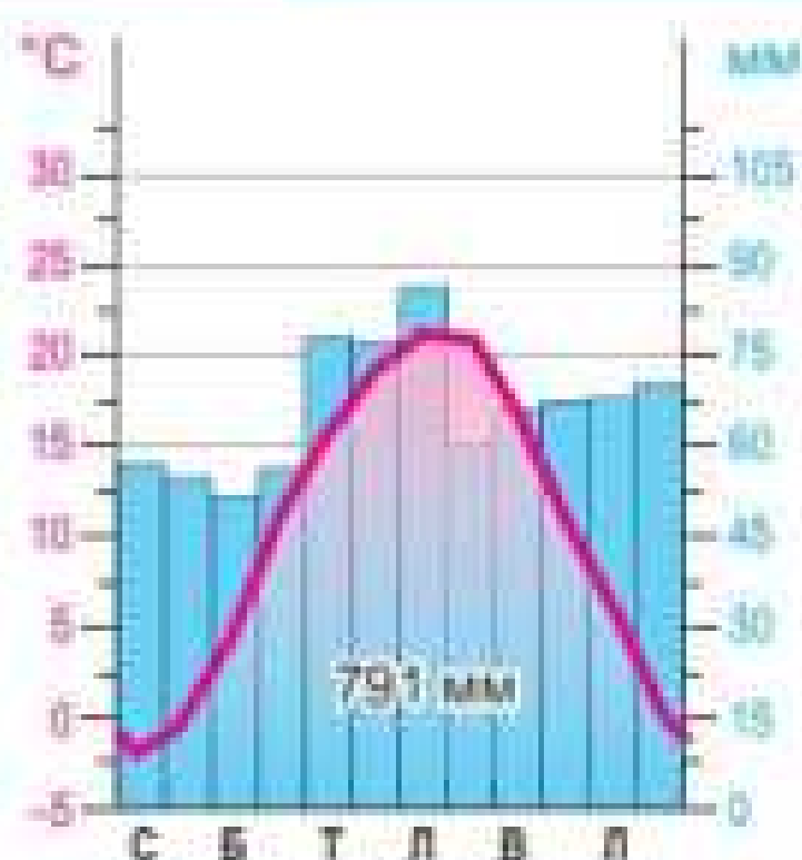
Мал. 104. Кліматодіаграма м. Ужгород
