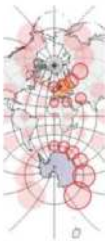
Мал. 22. Рівнокутна проєкція
