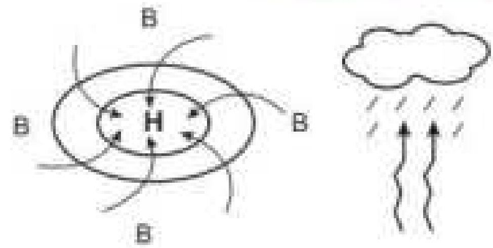
Мал. 99. Формування циклонів у Північній півкулі
