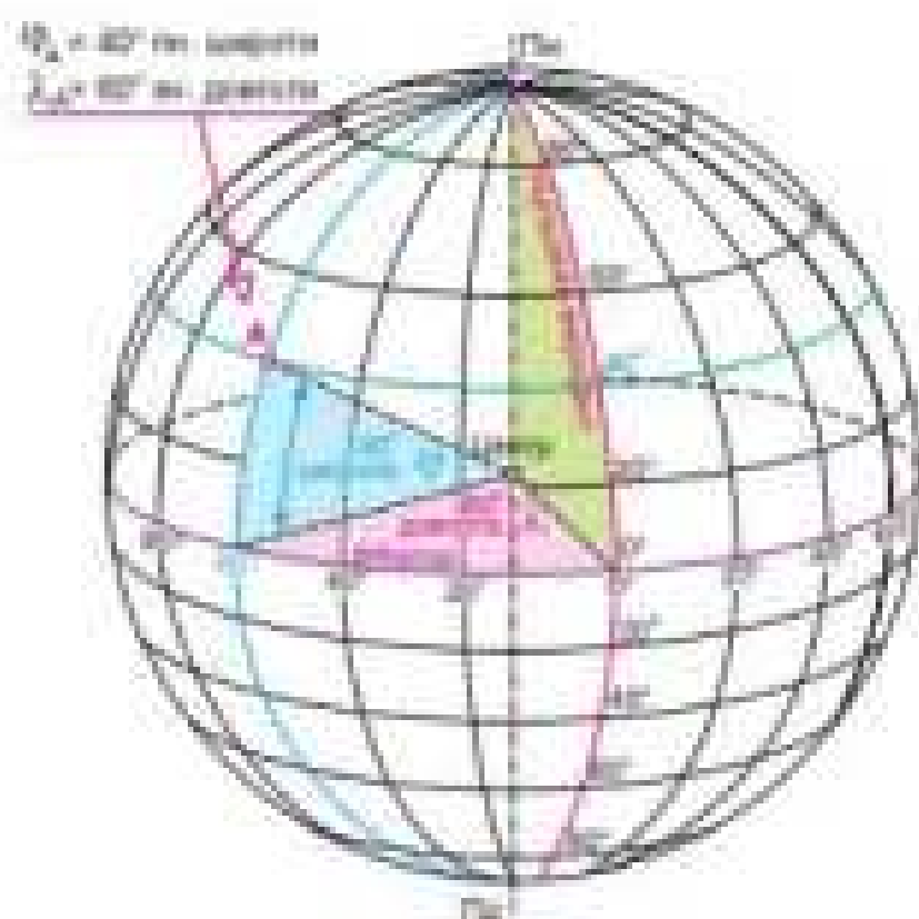
Мал. 31. Географічна система координат
