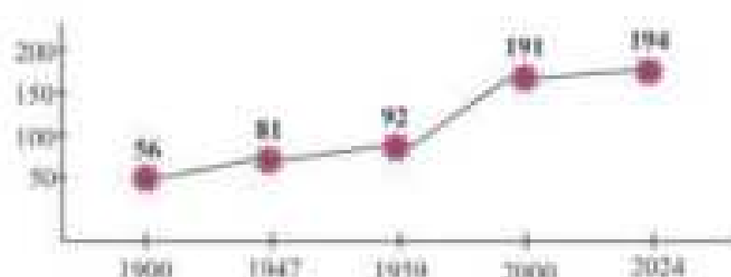
Мал. 50. Динаміка кількості держав у світі
