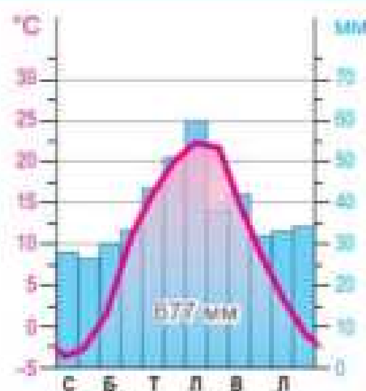
Мал. 106. Кліматодіаграма м. Київ
