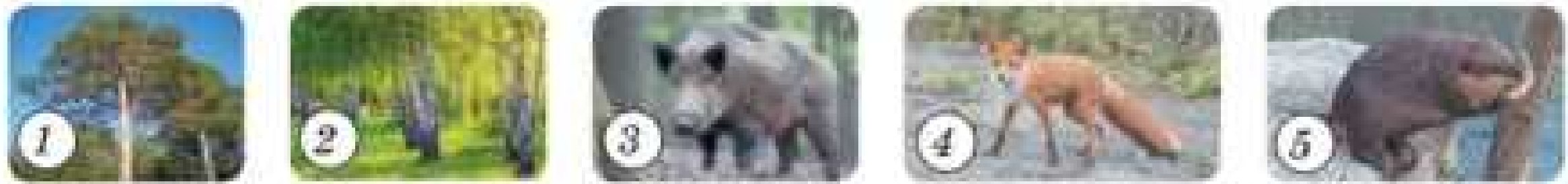
Мал. 161. Типові рослини і тварини Полісся: 1 – сосна; 2 – береза, 3 – кабан, 4 – лисиця, 5 – бобер
