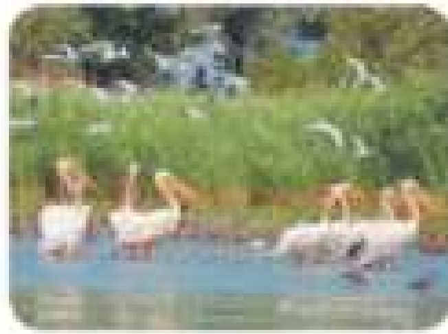
Мал. 187. Дунайський заповідник
