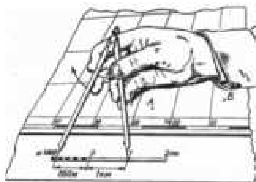
Мал. 44. Визначення відстані за допомогою циркуля-вимірника
