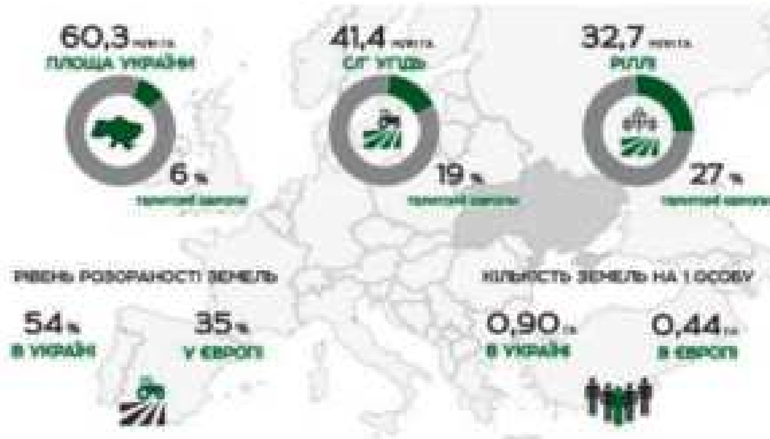
Мал. 146. Загальні дані про земельний фонд України
