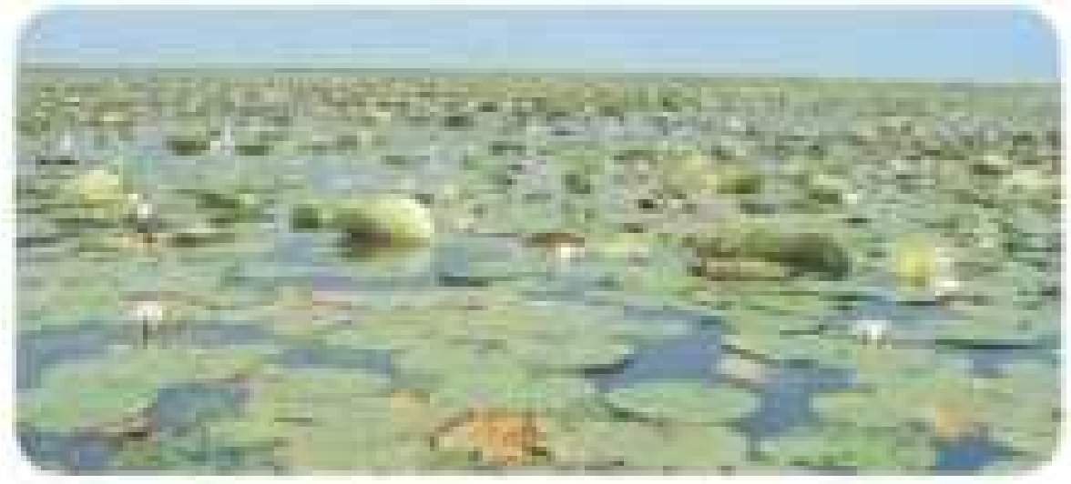
Мал. 152. Латаття дельти Дунаю
