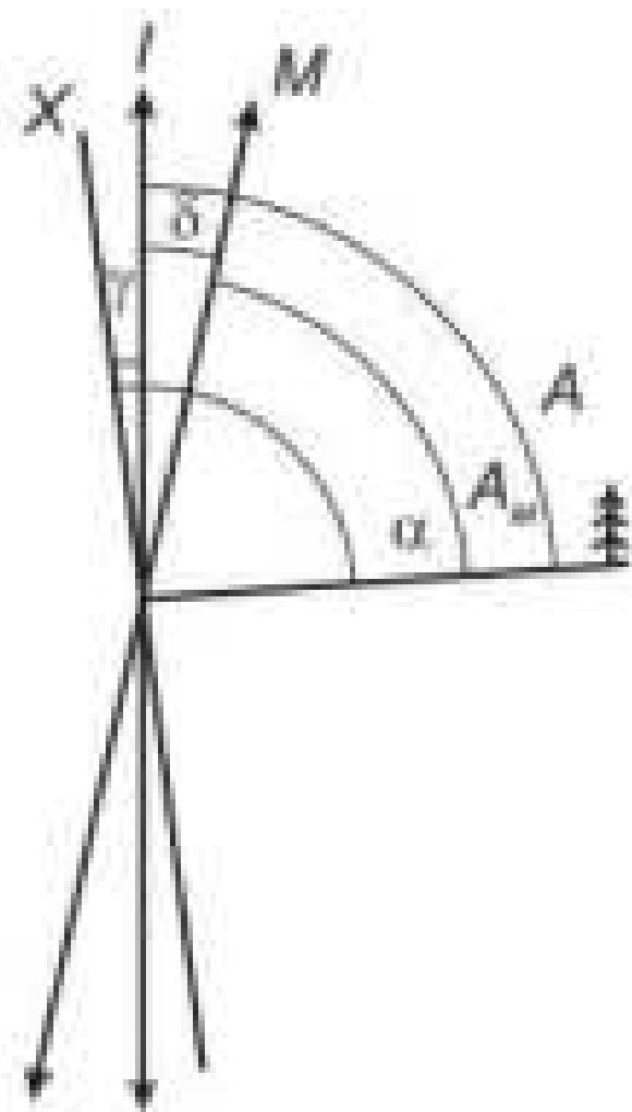
Мал. 37. Вимірювання кутів на топографічній карті
