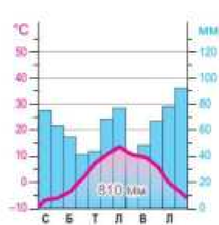
Мал. 108. Кліматодіаграма г. Роман-Кош
