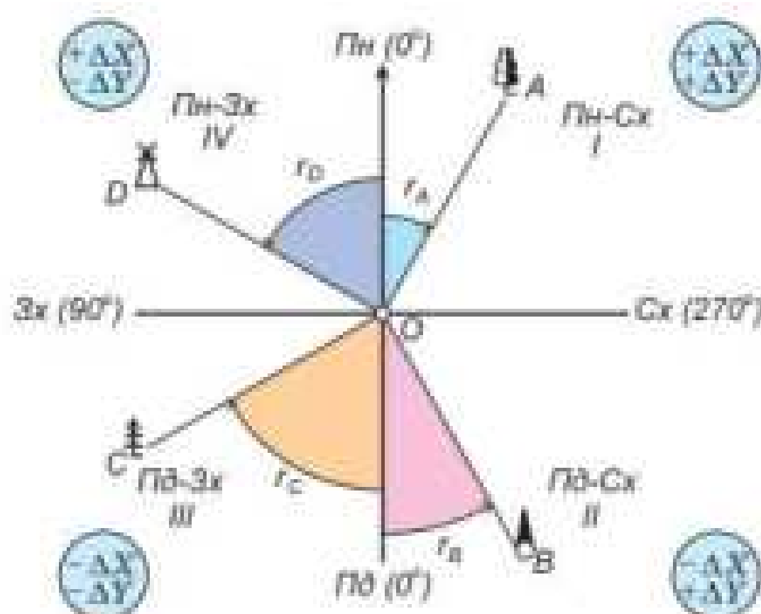
Мал. 42. Румби напрямків
