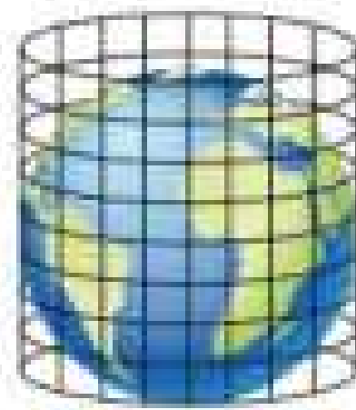
Мал. 20. Циліндрична проєкція
