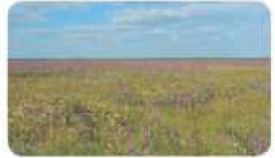
Мал. 169. Степовий ландшафт Дніпропетровщини
