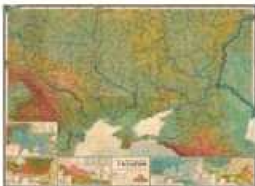
Мал. 13. Фізична карта України С. Рудницького масштабу 1:1 000 000 (Відень, 1918)
