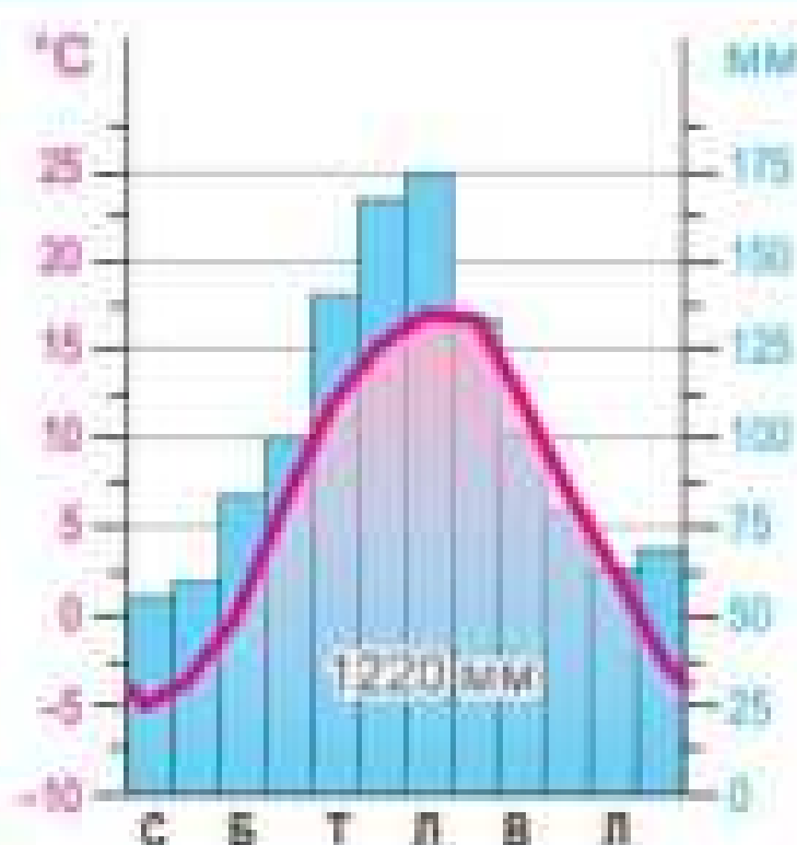
Мал. 105. Кліматодіаграма м. Яремче
