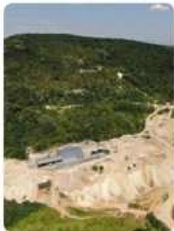
Мал. 91. Мужіївське родовище золота в Закарпатській обл.
