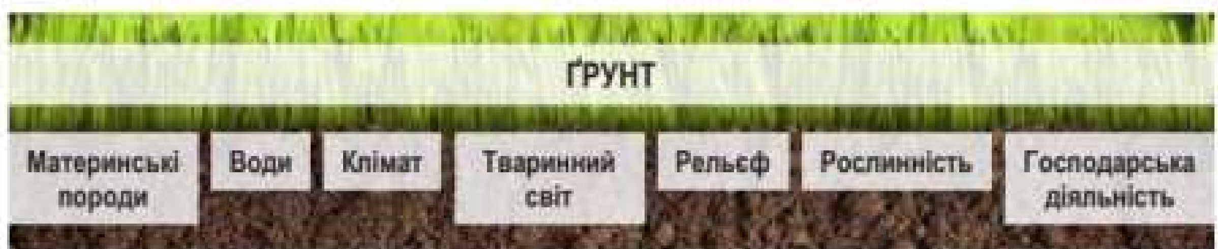
Мал. 142. Ґрунтоутворювальні чинники
