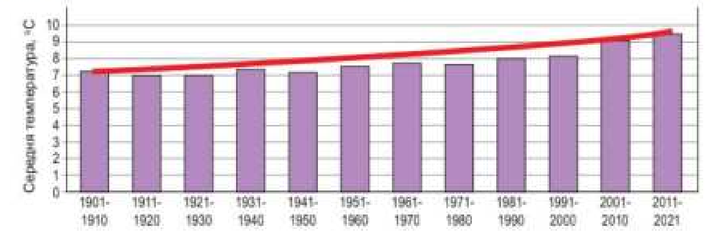
Мал. 115. Динаміка середньорічної температури в Україні
