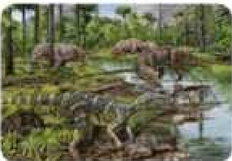
Мал. 75. Розвиток життя на Землі в періоди Мезозою
