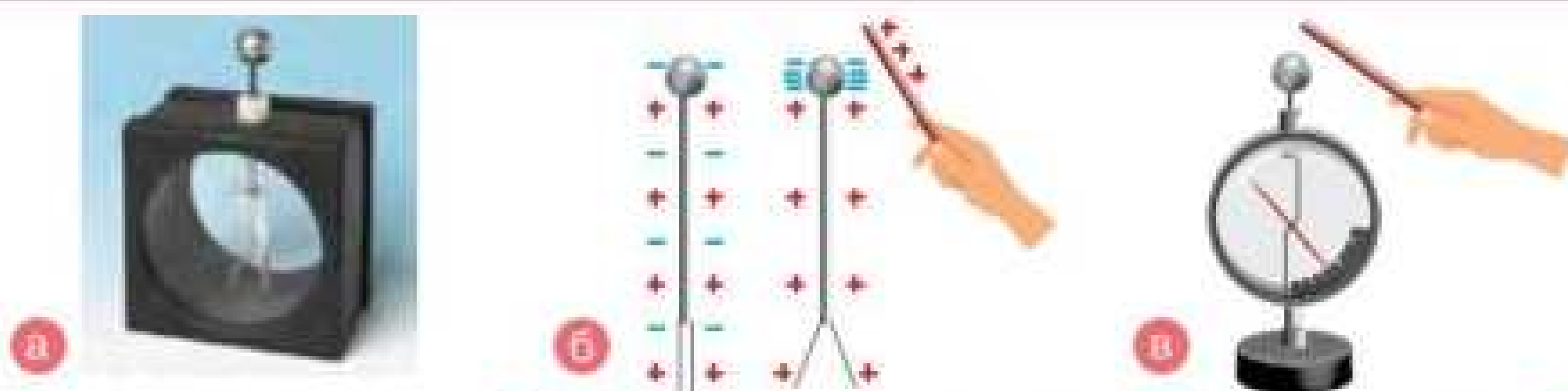
Мал. 19.6. Електроскоп (а), принцип дії електроскопа (б), електрометр (в)
