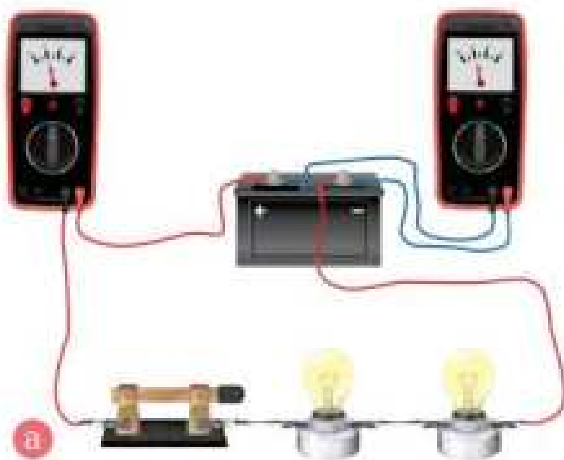
Мал. 27.2. Вимірювання напруги в колі з послідовним з'єднанням провідників:
