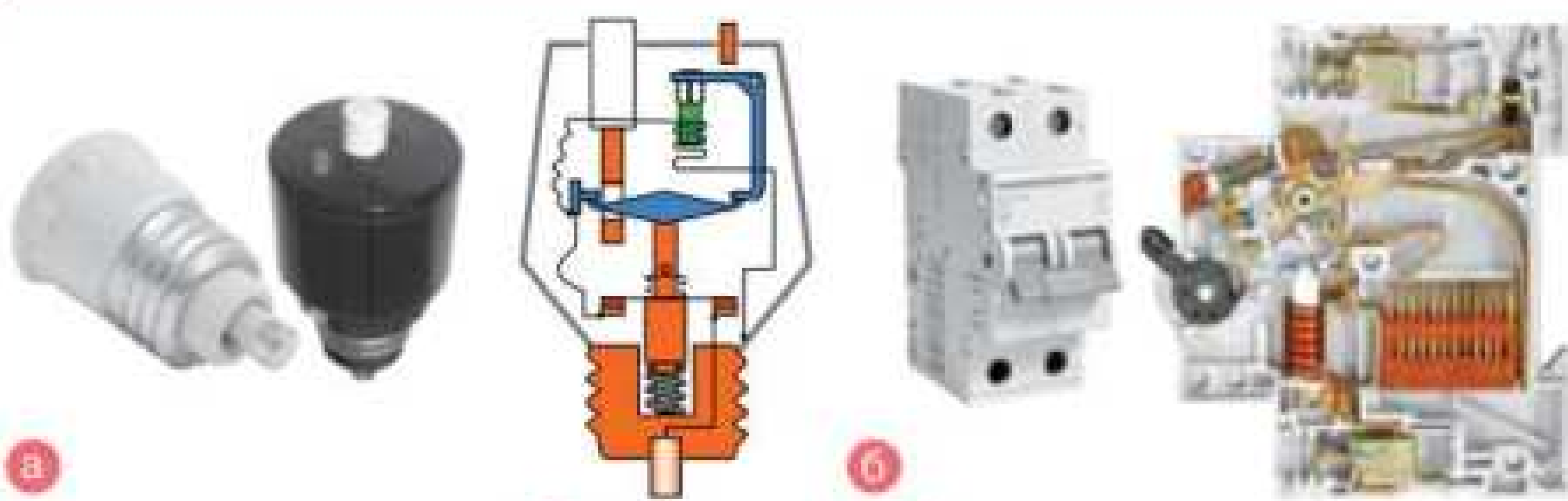
Мал. 32.4. Запобіжники: а — одноразові, б — автоматичні (багаторазові)
