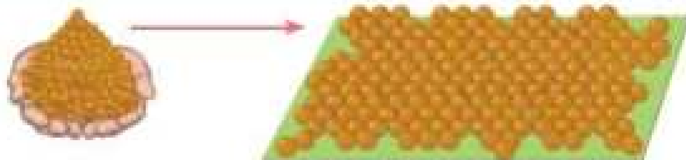
Мал. 1.9. Моделювання молекулярного шару
