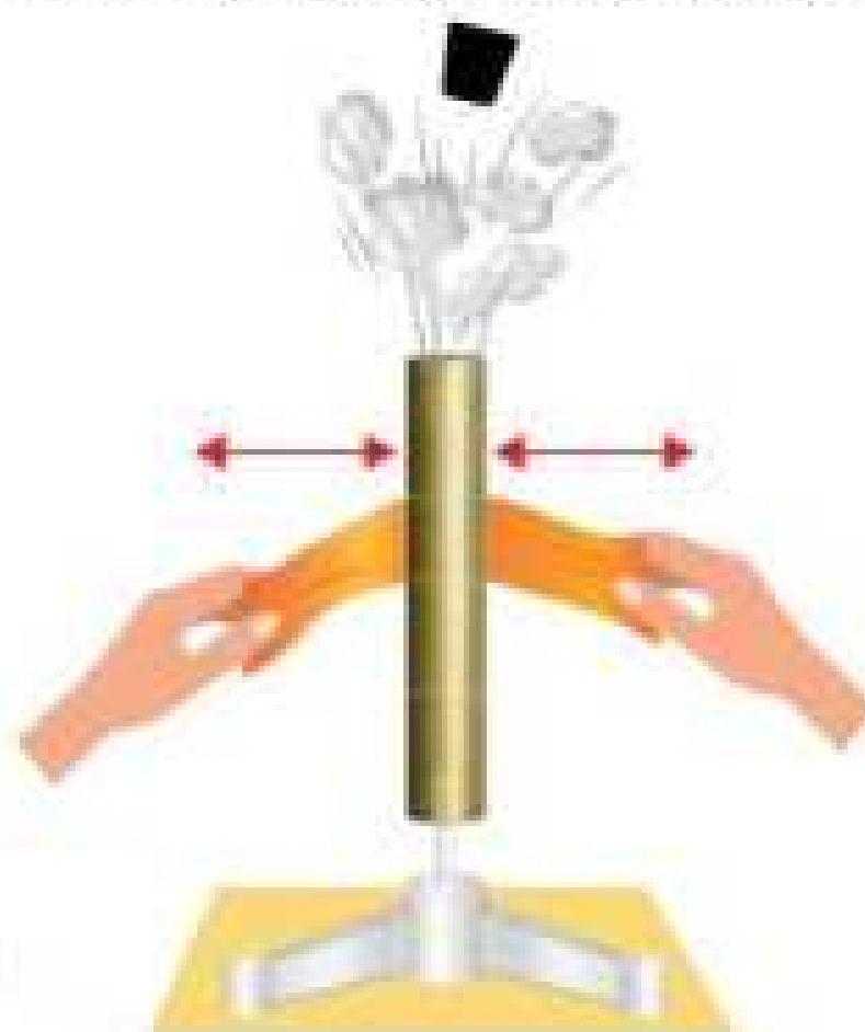
Мал. 5.2. Що є причиною зміни внутрішньої енергії у кожному випадку?
