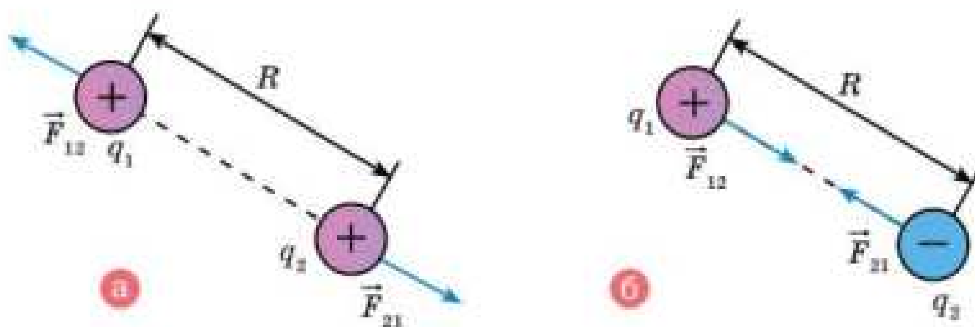
Мал. 20.3. Напрямки сил взаємодії точкових зарядів: а — однойменних; б — різнойменних
