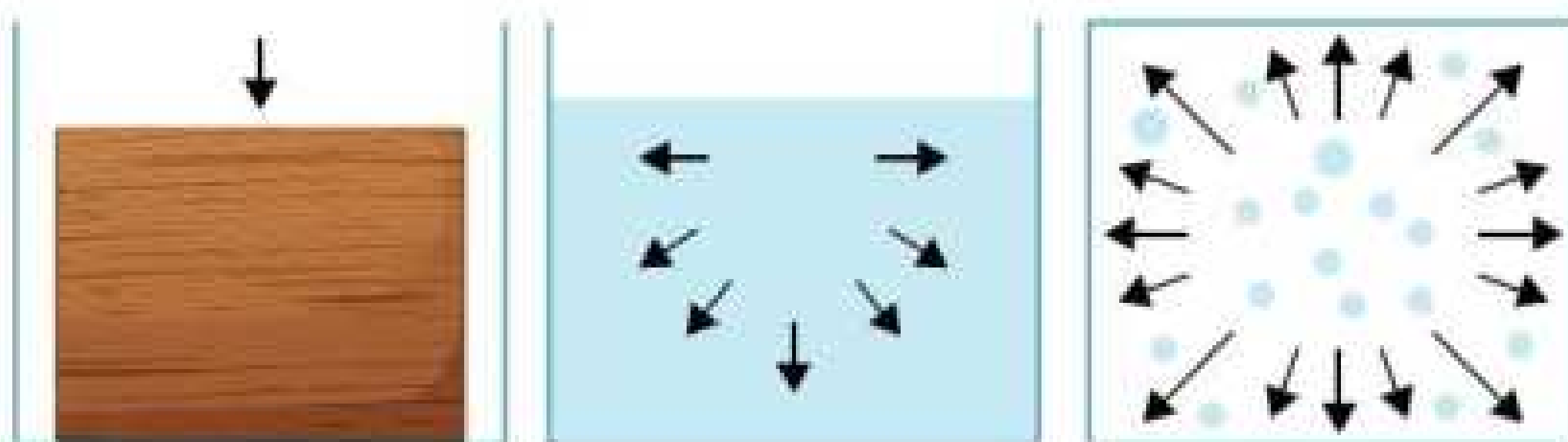
Мал. 2.3. Передавання тиску залежить від руху і взаємодії частинок речовини у різних агрегатних станах
