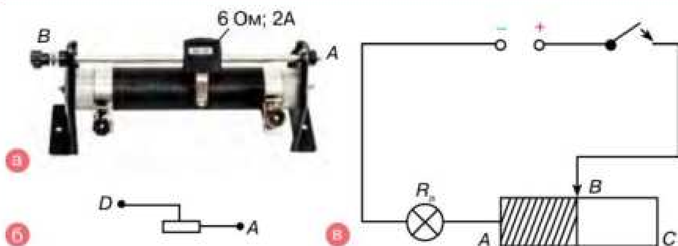
Мал. 25.6. Реостат: а — зовнішній вигляд, б — умовне зображення, в — схема роботи
