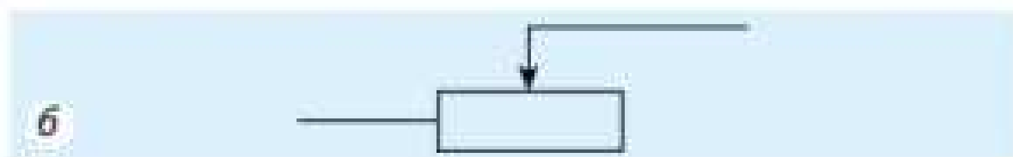
Рис. 38.3. Двоконтактний повзунковий реостат: а — загальний вигляд; 1, 6 — клеми; 2 — керамічний циліндр; 3 — металевий дріт (обмотка); 4 — повзунок; 5 — металевий стрижень; б — умовне позначення на схемах
