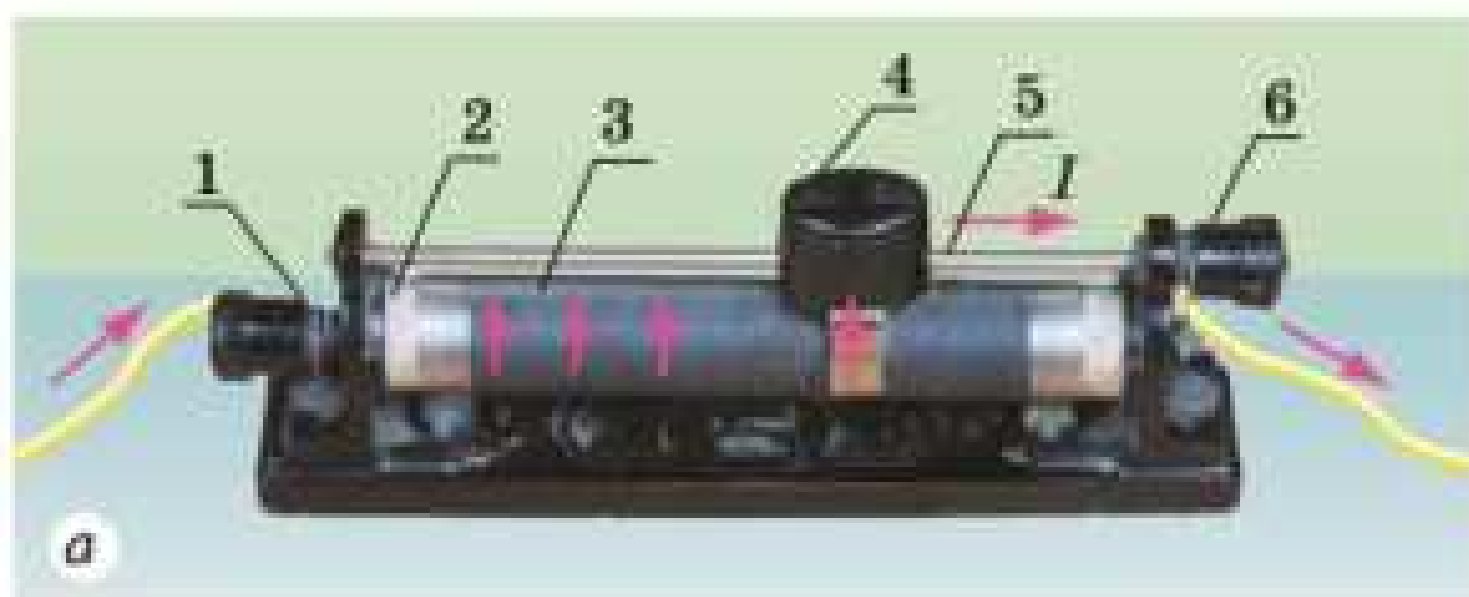
Рис. 38.3. Двоконтактний повзунковий реостат: а — загальний вигляд; 1, 6 — клеми; 2 — керамічний циліндр; 3 — металевий дріт (обмотка); 4 — повзунок; 5 — металевий стрижень; б — умовне позначення на схемах
