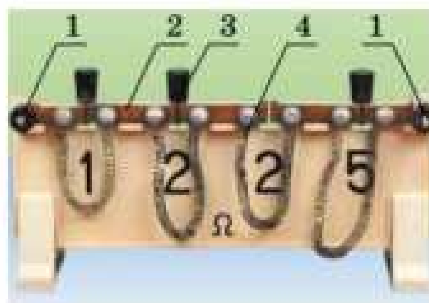
Рис. 4. Штепсельний реостат (магазин опорів): 1 — затискачі; 2 — мідна пластина; 3 — штепель; 4 — спіраль
