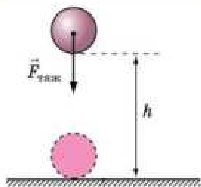
Рис. 7.3. Шлях l , який подолато тіло, що падало під дією сили тяжіння \vec{F}_{\text{тяж}} , дорівнює висоті h , на якій перебувало тіло
