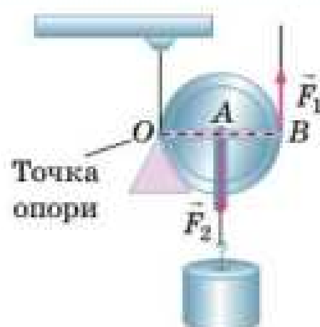
Рис. 3.4. Рухомий блок можна розглядати як важіль із відношенням плечей 1:2
