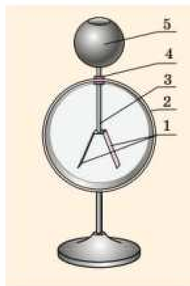
Рис. 29.6. Будова електроскопа: 1 — індикатор (паперові смужки); 2 — корпус; 3 — металевий стрижень; 4 — діелектрик; 5 — кондуктор
