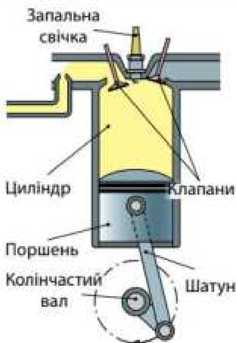
Рис. 25.2. Схема будови найпростішого двигуна внутрішнього згоряння
