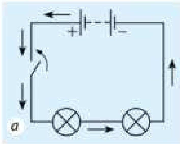
Рис. 34.4. Схеми деяких електричних кіл: а — схема послідовного з'єднання двох ламп (див. рис. 34.3, а); б — схема паралельного з'єднання двох ламп (див. рис. 34.3, б). Стрілками позначено напрямок струму в разі замкнення ключа
