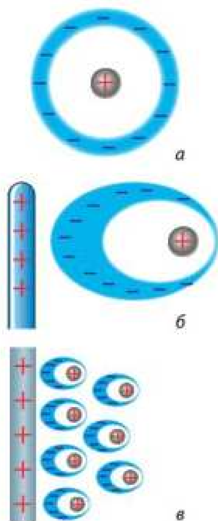
Рис. 29.5. Форма електронної хмари: за відсутності поля (а); за наявності поля (б). На поверхні паперу, ближчій до позитивно зарядженої палички, утворюється негативний заряд (в)
