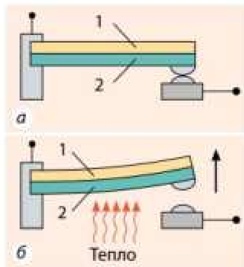
Рис. 11.4. Для автоматичного вимкнення електронагрівальних пристроїв (наприклад, чайника) використовують біметалеві пластинки (а). У разі збільшення температури металева смуга 2 розширюється більше, ніж смуга 1, виготовлена з іншого металу, тому пластинка вигинається і розмикає електричне коло (б)
