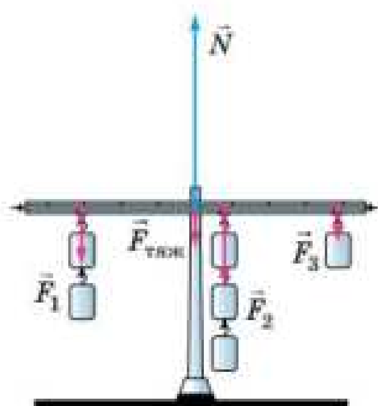
Рис. 2.3. Важіль залишається нерухомим, якщо справджується правило моментів і сили, що діють на важіль, скомпенсовані
