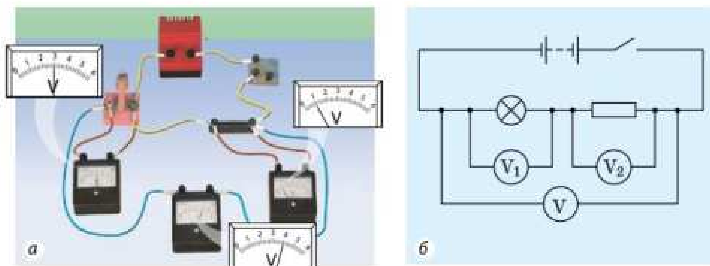
Рис. 39.3. Вимірювання напруги на різних ділянках електричного кола, яке складене з послідовно з'єднаних провідників: а — загальний вигляд електричного кола; б — схема. Загальна напруга на ділянці кола, яка містить послідовно з'єднані лампу та резистор, дорівнює сумі напруги на лампі та напруги на резисторі
