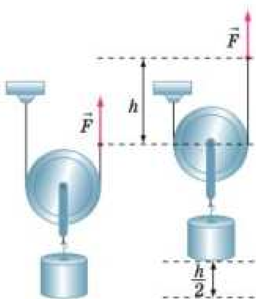
Рис. 3.5. Щоб за допомогою рухомого блоку підняти вантаж на висоту \frac{h}{2} , вільний кінець мотузки слід підняти на висоту h
