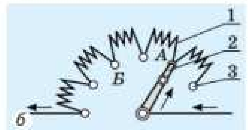
Рис. 38.4. Важільний (секційний) реостат: а — загальний вигляд; б — схема: 1 — металевий дріт; 2 — важіль; 3 — контакт; стрілками показано напрямки струму
