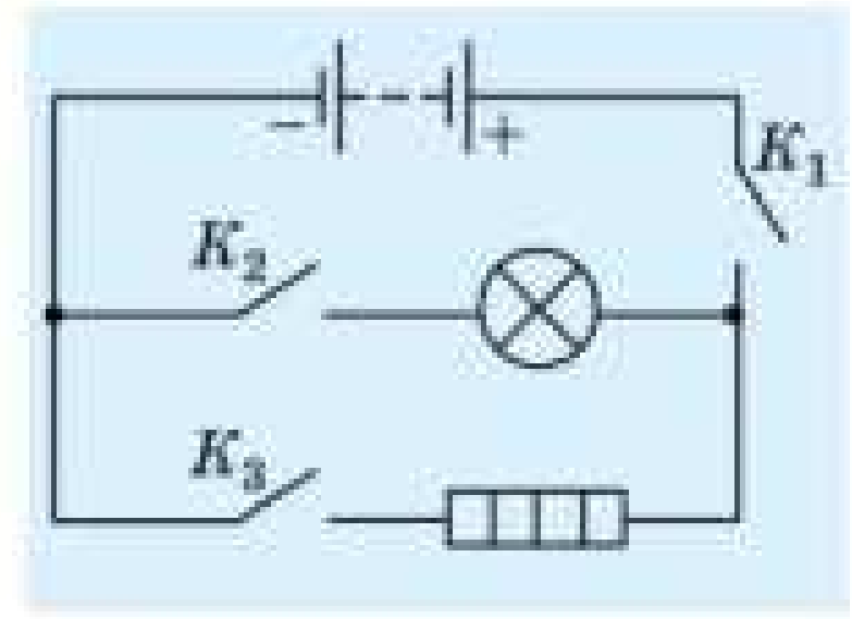
Рис. 34.5. Схема вмикання електричної лампи та обігрівача
