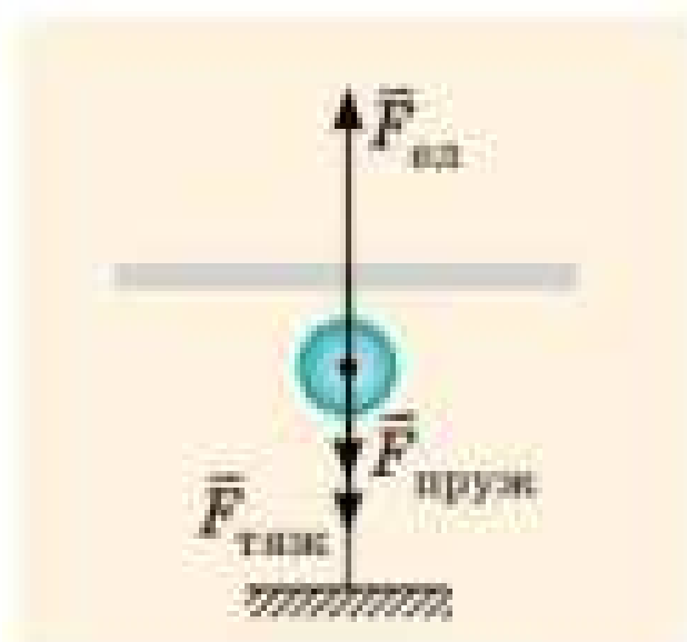
Рис. 28.1. Негативно заряджена кулька притягується до позитивно зарядженої пластини з оргскла. Кулька перебуватиме в спокої, коли сили тяжіння \vec{F}_{\text{тяж}} і натягу нитки \vec{F}_{\text{пруж}} скомпенсовані силою \vec{F}_{\text{ел}} , яка діє на кульку з боку наелектризованої пластини
