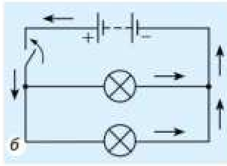
Рис. 34.4. Схеми деяких електричних кіл: а — схема послідовного з'єднання двох ламп (див. рис. 34.3, а); б — схема паралельного з'єднання двох ламп (див. рис. 34.3, б). Стрілками позначено напрямок струму в разі замкнення ключа
