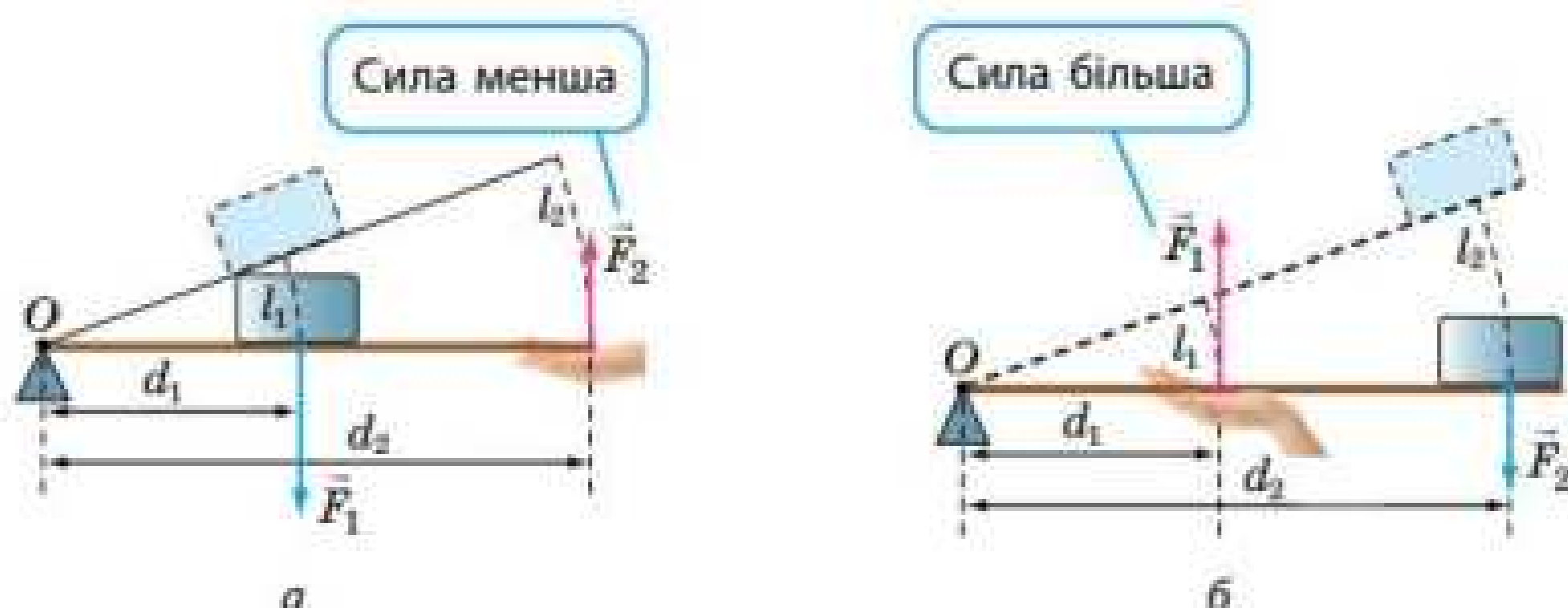
Рис. 2.4. За допомогою важеля можна отримати як виграш у силі (а), так і виграш у відстані (б): точка прикладання меншої сили ( \vec{F}_2 ) завжди проходить більший шлях ( l_2 ), а точка прикладання більшої сили ( \vec{F}_1 ) — менший шлях ( l_1 )
