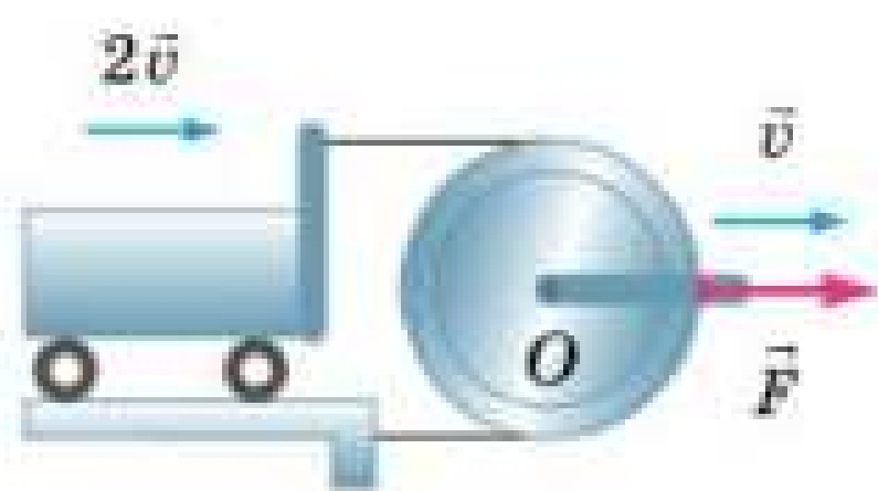
Рис. 3.6. Якщо точку прикладання сили \vec{F} переміщувати з певною швидкістю \vec{v} , то візок рухатиметься удвічі швидше
