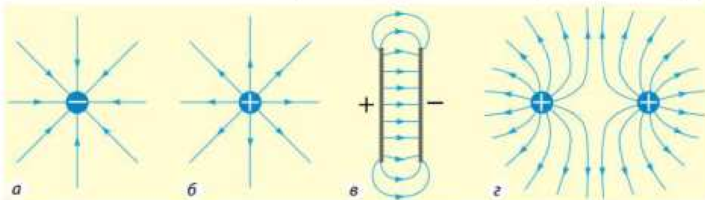
Рис. 28.6. Картини силових ліній електричних полів, створених: а — негативно зарядженою кулькою; б — позитивно зарядженою кулькою; в — системою двох паралельних пластин, заряди яких однакові за модулем і протилежні за знаком; г — системою двох кульок, що мають однакові позитивні заряди
