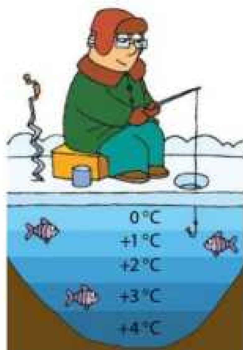
Рис. 11.3. Розподіл температур у глибокій водоймі взимку. Найвища температура води — на дні водойми, найнижча ( 0^{\circ}\text{C} ) — безпосередньо під шаром льоду
