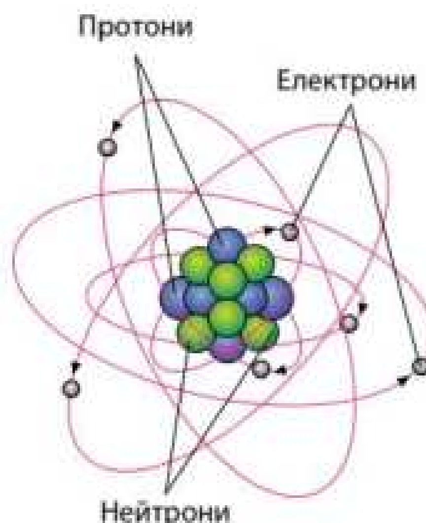
Рис. 27.4. Електрони і протони разом з електронейтральними нейтронами є складовими атомів, з яких побудовані речовини
