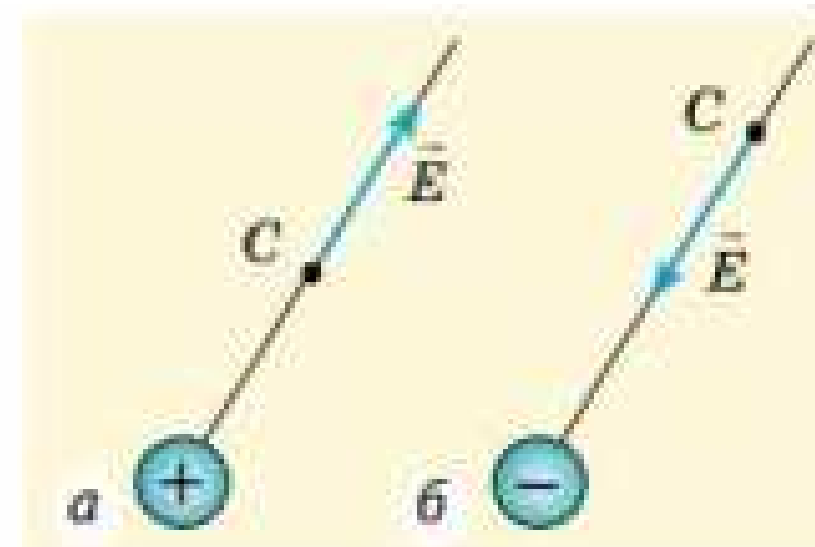
Рис. 28.4. Визначення напрямку напруженості \vec{E} електричного поля в точці С
