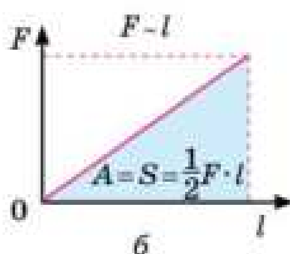
Рис. 4.2. Площа S фігури під графіком залежності сили F від шляху l чисельно дорівнює роботі сили
