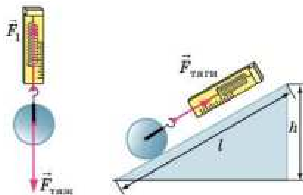
Рис. 6.2. Корисна робота — це те, що нам потрібно зробити (підняти тіло); повна робота — це те, як ми це робимо (тягнемо похилою площиною)
