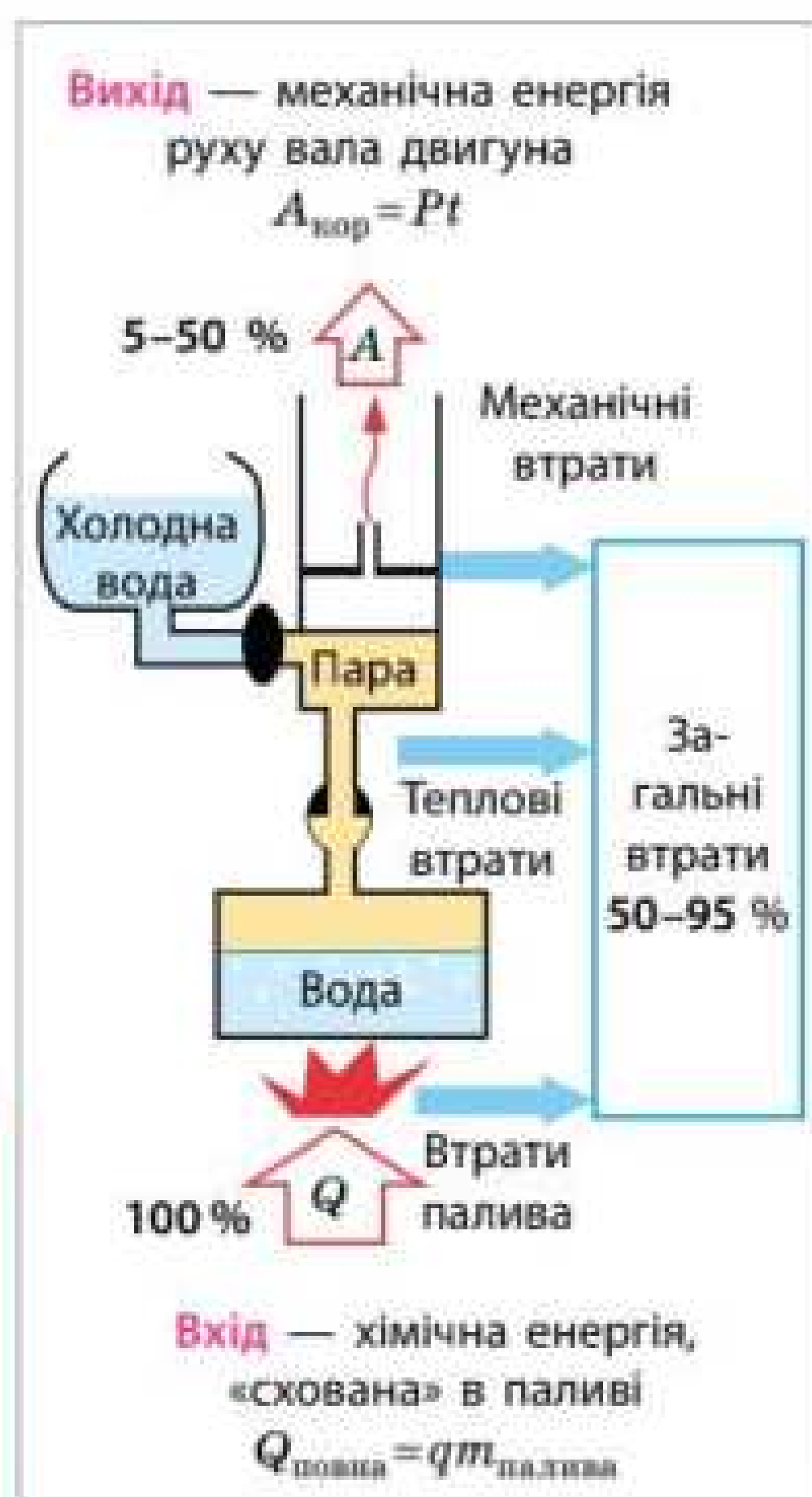
Рис. 24.3. ККД парових теплових двигунів і схема втрат енергії
