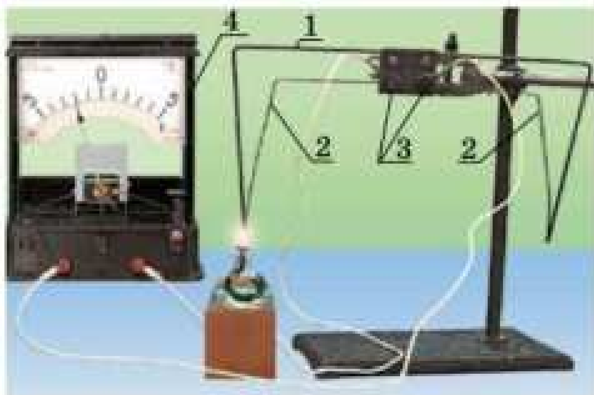
Рис. 33.4. Термопара — пристрій для перетворення теплової енергії на електричну. До кінців константового дроту (1) припаяно два залізні дроти (2), вільні кінці яких (3) з'єднані з гальванометром* (4). Якщо нагріти місце спая, гальванометр зафіксує наявність струму
