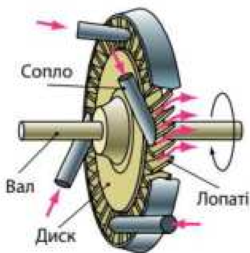
Рис. 25.1. Схема будови найпростішої парової турбіни
