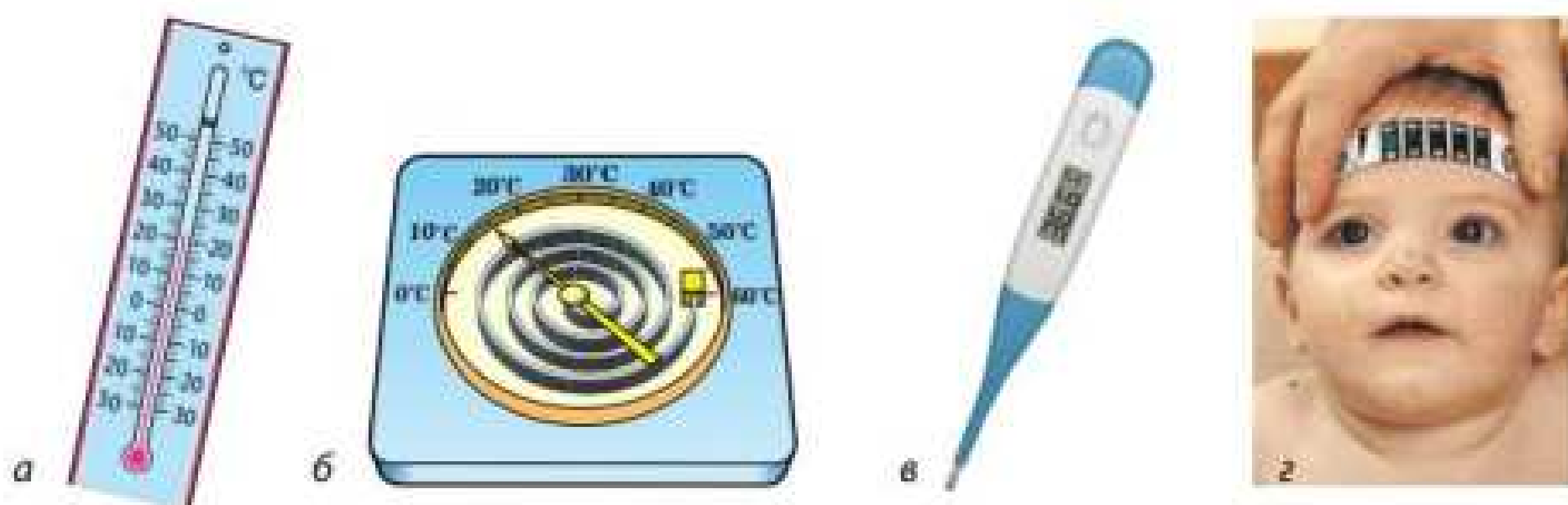
Рис. 10.3. Різні види термометрів: а — рідинний (мірою температури є довжина стовпчика рідини); б — біметалевий (біметалева пластинка, яка з'єднана зі стрілкою термометра, вигинається в результаті нагрівання); в — побутовий електронний термометр (зі зміною температури змінюються покази на цифровому табло); г — рідинно-кристалічний (унаслідок зміни температури змінюється колір відповідної ділянки термометра)
