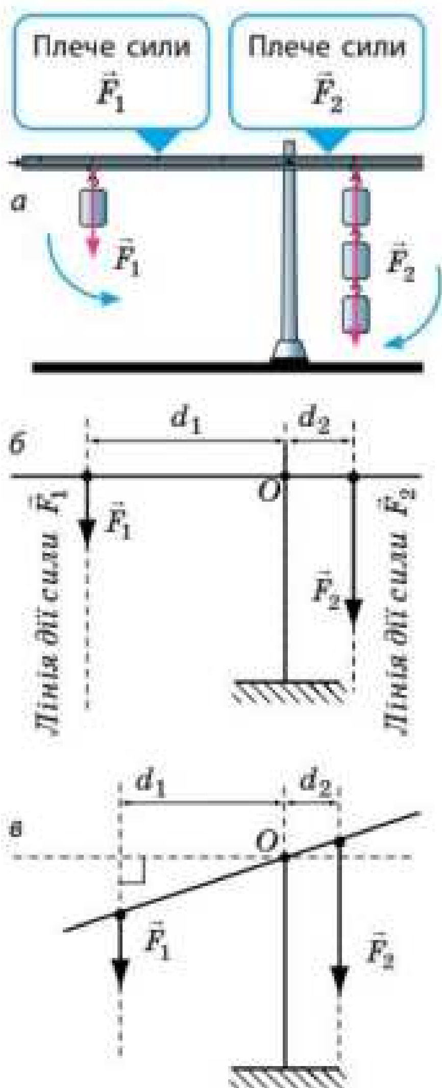
Рис. 2.2. Щоб знайти плече сили, слід від точки опори провести перпендикуляр до лінії дії сили. Тут O — точка опори; d_1 — плече сили \vec{F}_1 ; d_2 — плече сили \vec{F}_2
