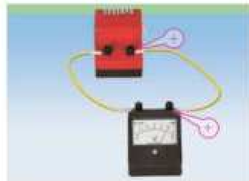
Рис. 36.3. Вимірювання вольтметром напруги на виході джерела струму
