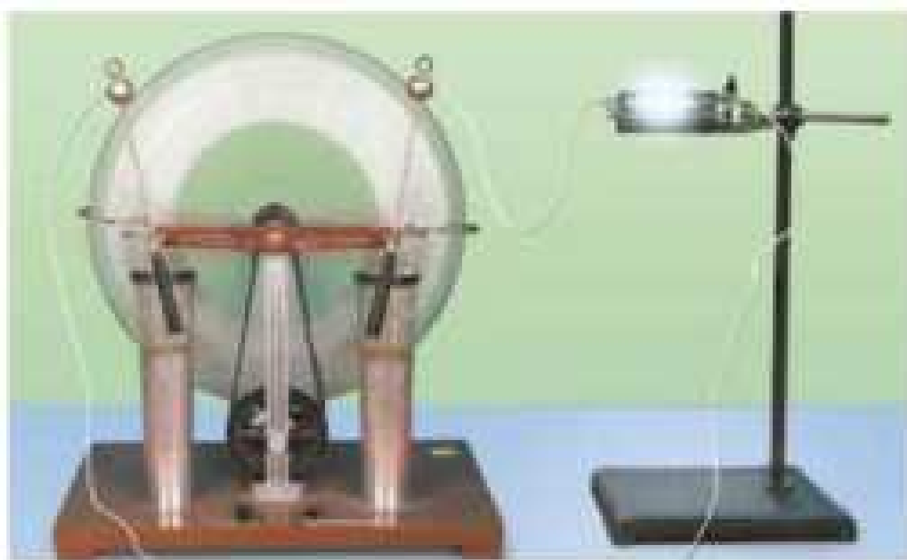
Рис. 33.2. Якщо різнойменно заряджені кондуктори електрофорної машини з'єднати з електричною лампою, у лампі виникне електричний струм. Лампа світитиметься, поки обертаються диски машини, — у цьому випадку механічна енергія перетворюється на електричну
