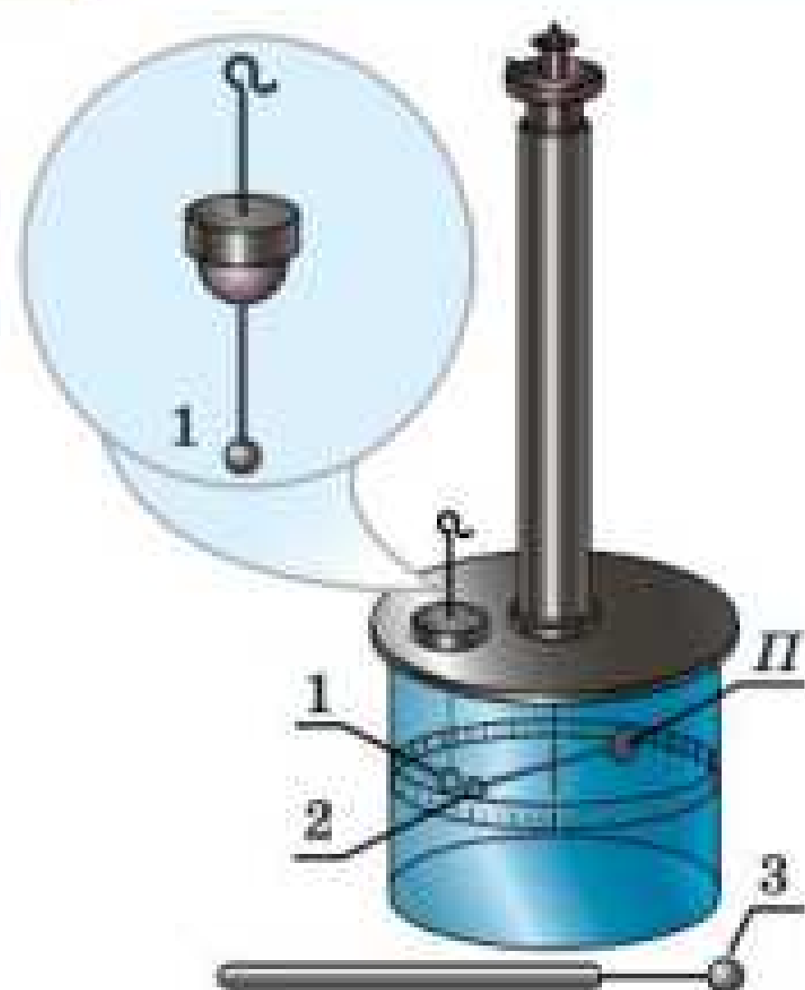
Рис. 30.2. Крутильні терези Кулона. На металевому дроті закріплене коромисло, на кінцях якого розміщені кулька 2 і протизвага П. Крізь отвір у кришці скляного циліндра опускають кульку 1. Кулька 3 розташована на тримачі, який виготовлений із діелектрика
