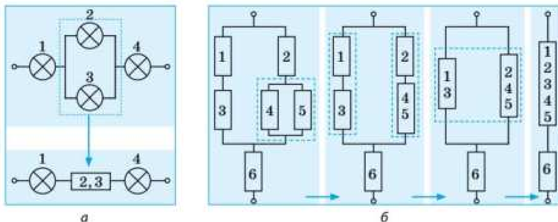
Рис. 40.5. Приклади покрокового спрощення електричної схеми
