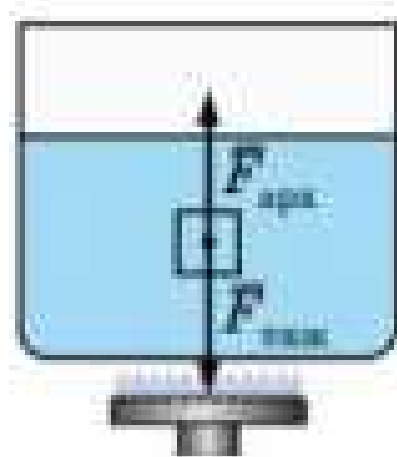
Рис. 14.3. На будь-який невеликий об'єм рідини діють сила тяжіння та виштовхувальна (архімедова) сила
