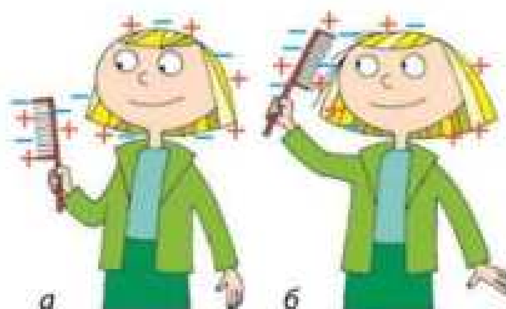
Рис. 29.2. Перед розчісуванням кількість позитивних зарядів на волоссі й гребінці дорівнює кількості негативних (а). Під час розчісування частина електронів з волосся перейде на гребінець, у результаті чого гребінець зарядиться негативно, а волосся — позитивно (б)
