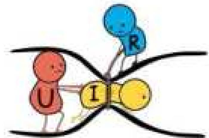
Рис. 37.5. Візуалізація закону Ома
