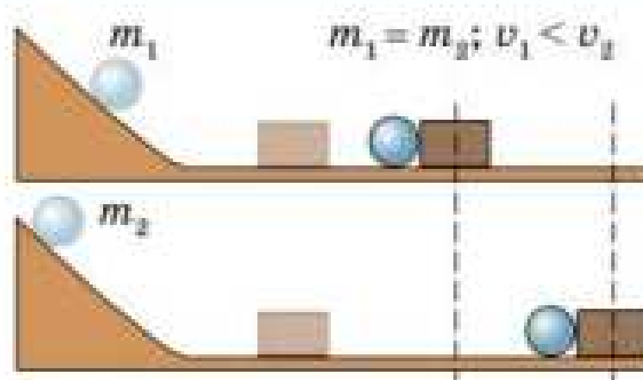
Рис. 7.7. Чим більшою є швидкість руху кулі, тим більшу кінетичну енергію має куля
