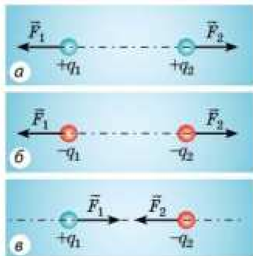
Рис. 30.3. Сили електричної взаємодії ( \vec{F}_1 і \vec{F}_2 ) напрямлені вздовж умовної прямої, яка з'єднує точкові заряди
