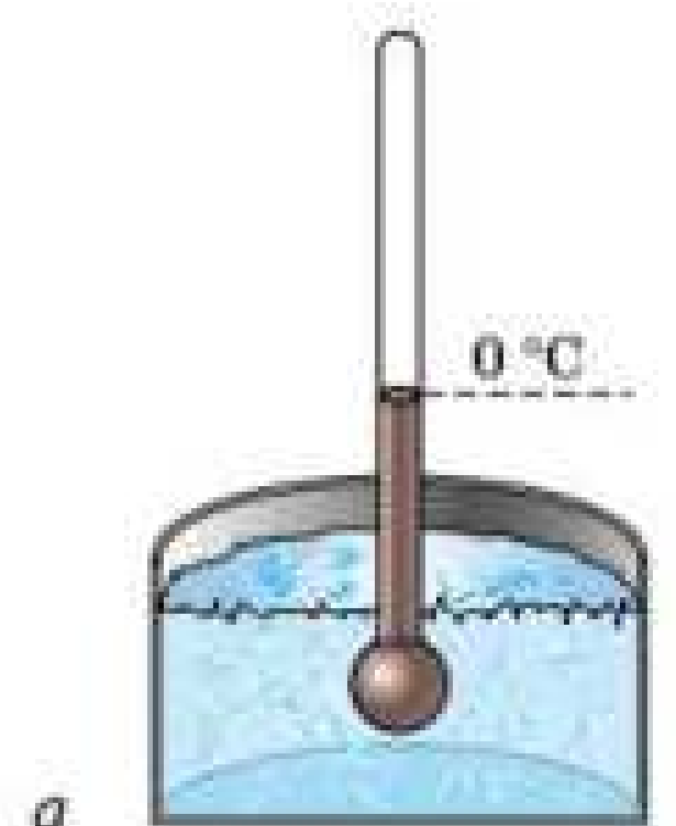
а Температурі танення льоду приписують значення 0^{\circ}\text{C}
