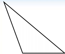
Тупокутний трикутник –
