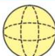
Куля
