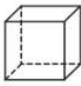
Гексаедр
