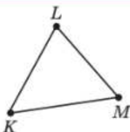
Трикутник
