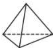
Тетраедр
