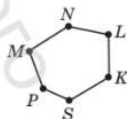
Шестикутник
