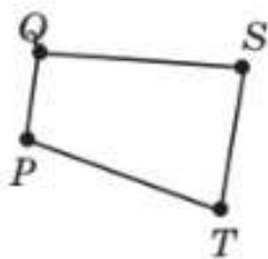
Чотирикутник
