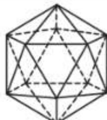
Ікосаедр
