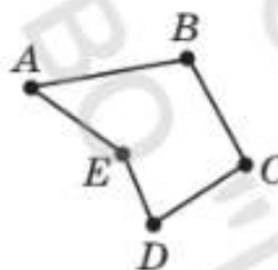
П'ятикутник
