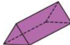
Трикутна призма
