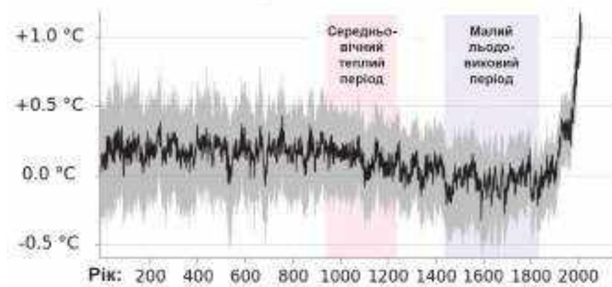
Графік глобальної температури за 2 тисячі років (так званий «Середньовічний теплий період» позначено рожевим, а «Малый льодовиковий період» — блакитним), графік Еда Хокінса, 2019 рік
