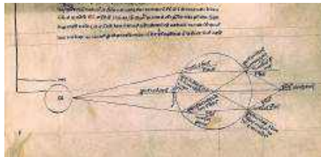
Заломлення світла сферичною склянню ємністю, наповненою водою, Роджер Бекон, «De multiplicacione specierum», XIII ст.
