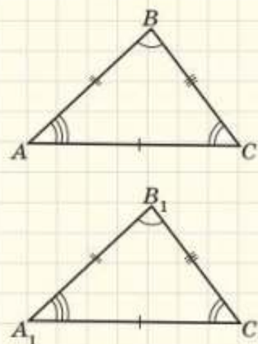
Рис. 56. Трикутники ABC і A_1B_1C_1 рівні
