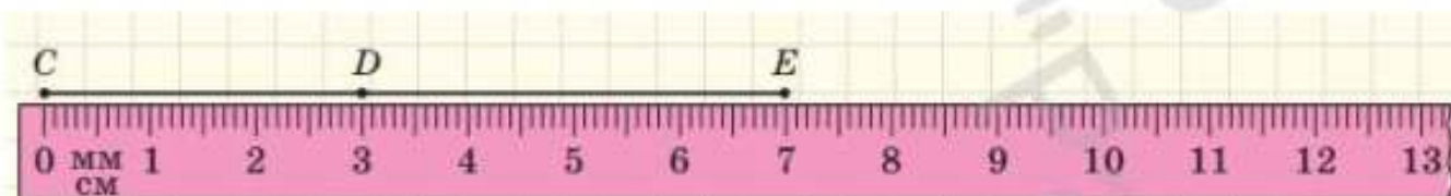
Рис. 15. Вимірювання відрізка за допомогою лінійки
