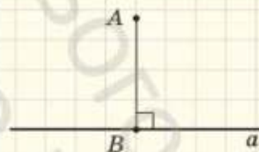
Рис. 70. Відрізок AB — перпендикуляр до прямої a
