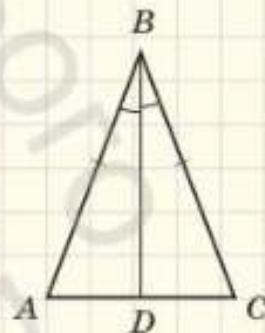
Рис. 83. Промінь BD — бісектриса кута B
