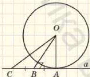
Рис. 168. До доведення властивості дотичної
