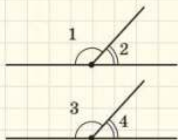
Рис. 39. Кути, суміжні з рівними кутами, також рівні
