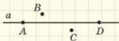
Рис. 1. Точки A і D лежать на прямій a , а точки B і C не лежать на прямій a
