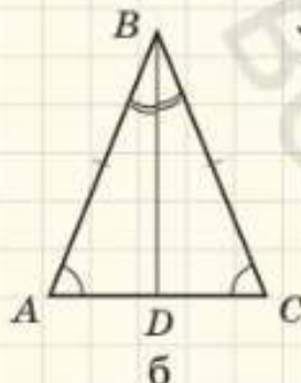
Рис. 101. Відрізок BD — медіана, бісектриса й висота рівнобедреного трикутника ABC
