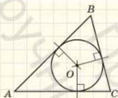
Рис. 186. Коло, вписане в трикутник ABC
