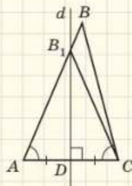
Рис. 85. До доведення ознаки рівнобедреного трикутника
