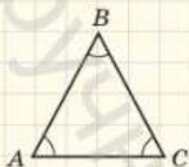
Рис. 86. До ознаки рівностороннього трикутника
