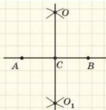
Рис. 172. Побудова середини відрізка
