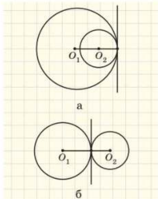
Рис. 171. Дотик двох кіл: а) внутрішній; б) зовнішній
