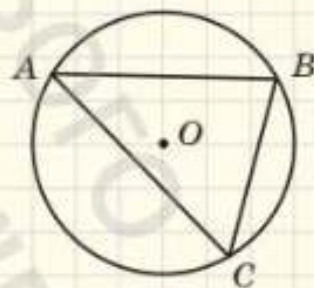
Рис. 183. Коло, описане навколо трикутника ABC
