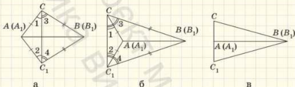
Рис. 107. Прикладання трикутника A_1B_1C_1 до трикутника ABC
