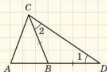
Рис. 157. До доведення нерівності трикутника
