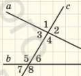
Рис. 118. Пряма c перетинає прямі a і b
