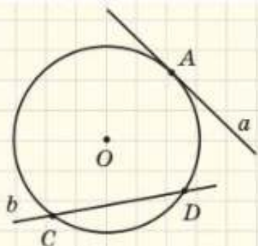
Рис. 167. Січна й дотична до кола
