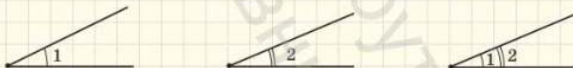
Рис. 20. Кути 1 і 2 суміщаються накладанням
