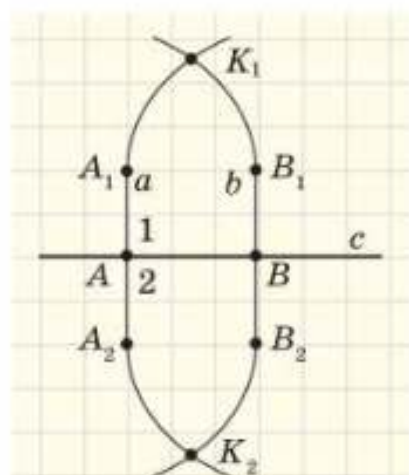
Рис. 50. До припущення про те, що прямі A_1A_2 і B_1B_2 перетинаються
