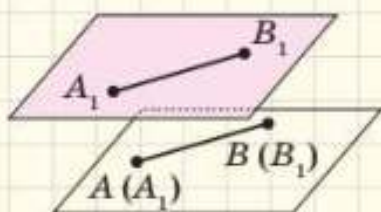
Рис. 12. Відрізки AB і A_1B_1 суміщаються накладанням
