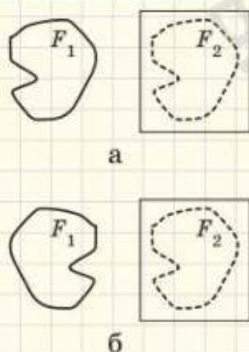
Рис. 55. Фігури F_1 і F_2 суміщаються накладанням
