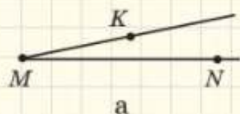
Рис. 8. До пояснення поняття «доповняльні промені»:
