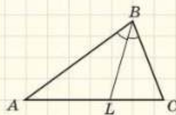
Рис. 97. Відрізок BL — бісектриса трикутника ABC
