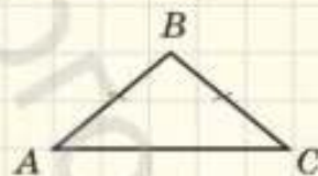
Рис. 81. Трикутник ABC — рівнобедрений з основою AC
