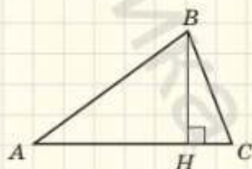
Рис. 99. Відрізок BH — висота трикутника ABC
