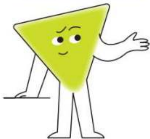
Рис. 156. До доведення співвідношення між сторонами і кутами трикутника
