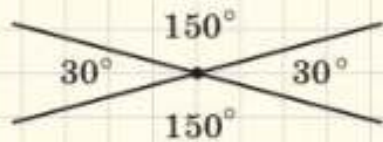
Рис. 47. Дві прямі перетинаються під кутом 30^\circ
