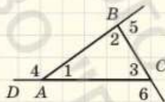
Рис. 146. Зовнішній кут 4 дорівнює сумі кутів 2 і 3
