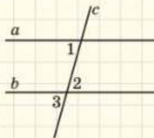
Рис. 121. \angle 1 = \angle 3 , тоді a \parallel b
