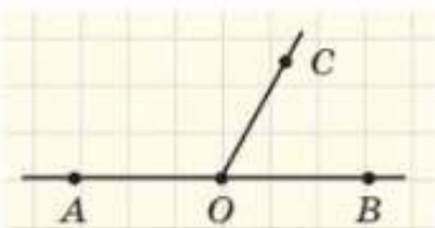
Рис. 35. Кути AOC і COB суміжні
