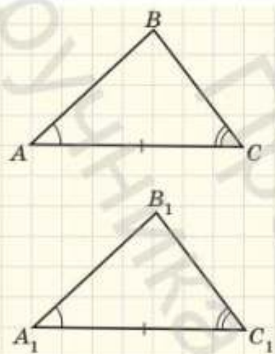
Рис. 72. Трикутники ABC і A_1B_1C_1 рівні за стороною та прилеглими до неї кутами
