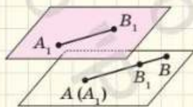
Рис. 13. Відрізки AB і A_1B_1 не суміщаються накладанням
