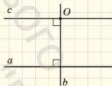
Рис. 173. Побудова прямої, паралельної даній
