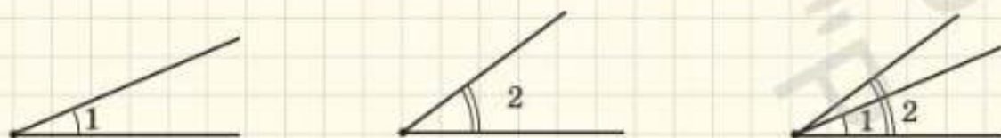
Рис. 21. Кути 1 і 2 не суміщаються накладанням
