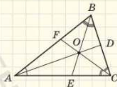
Рис. 187. Точка O — точка перетину бісектрис трикутника ABC
