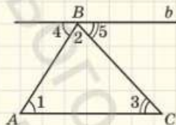
Рис. 141. До доведення теореми про суму кутів трикутника
