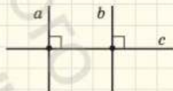
Рис. 49. Дві прямі, перпендикулярні до третьої, паралельні
