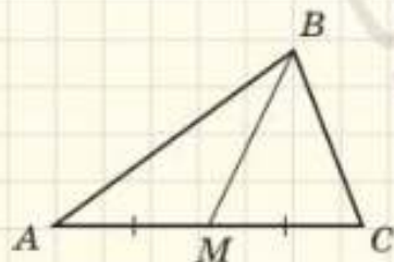
Рис. 95. Відрізок BM — медіана трикутника ABC
