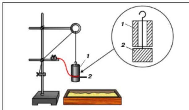
Мал. 87. Демонстрування невагомості тіла
