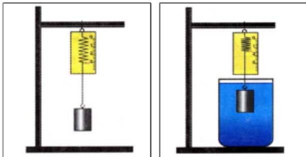
Мал. 104. Прилади для визначення густини твердого тіла.
