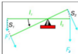
Мал. 130. Важіль не дає виграшу в роботі
