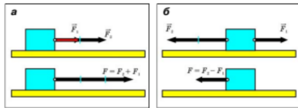
Мал. 82. Схема додавання сил, що діють уздовж однієї прямої
