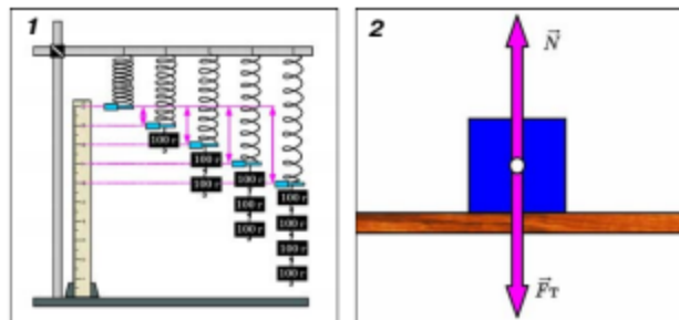
Мал. 69. Дія сили пружності: 1 — поступове розтягування пружини, 2 — вантаж на столі перебуває у спокої
