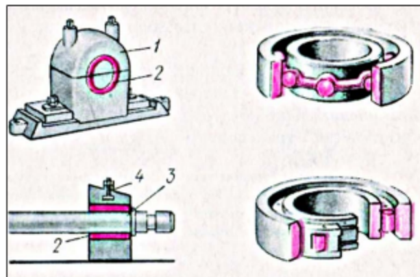
Мал. 91. Підшипники ковзання: 1 — корпус підшипника; 2 — вкладиш; 3 — вал; 4 — отвір для змащування
