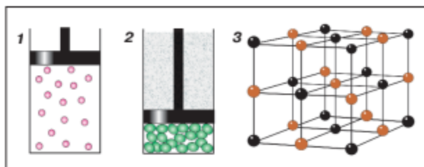
Мал. 11. 1 — газ; 2 — рідина; 3 — тверде тіло
