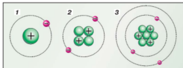
Мал. 8. Моделі атомів: 1 — Гідрогену; 2 — Гелію; 3 — Літію
