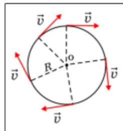
Мал. 42. Напрямок швидкості під час руху тіла по колу
