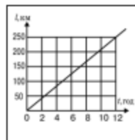
Мал. 36. До задачі 2
