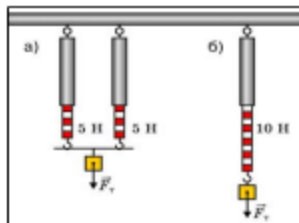
Мал. 79. Дія сил в одному напрямку
