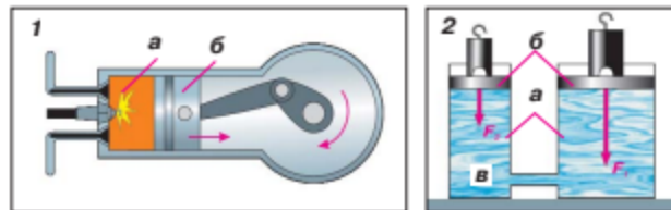
Мал. 19. 1 — модель двигуна: а — камера згорання, б — поршень; 2 — модель гідравлічного преса: а — циліндри, б — поршні, в — рідина
