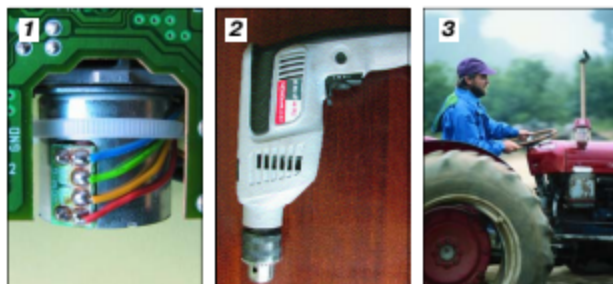
Мал. 108. Двигуни різної потужності: 1 – двигун у комп’ютерній техніці (0,1 Вт); 2 – двигун електродрелі (780 Вт); 3 – двигун трактора (50 кВт)
