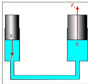
Мал. 98. Модель гідравлічного преса
