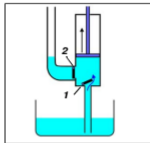
Мал. 100. Рідинний насос
