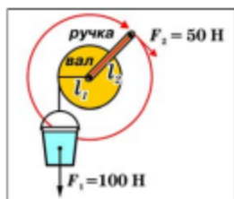
Мал. 116. Коловорот
