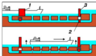
Мал. 97. Річковий шлюз в сполучених посудинах
