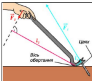
Мал. 128. Цяховиймач
