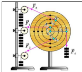
Мал. 125. Прилад для визначення умови рівноваги тіла, що має вісь обертання
