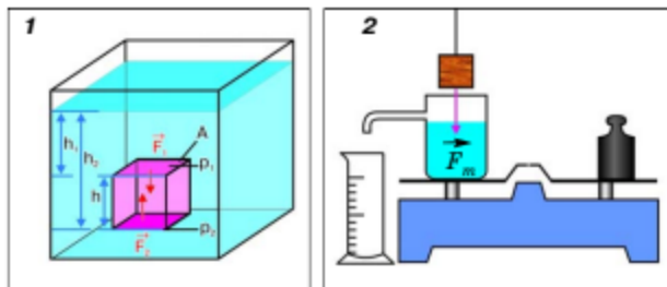
Мал. 103. 1 — дія сил на занурене у рідину тіло; 2 — до задачі 1
