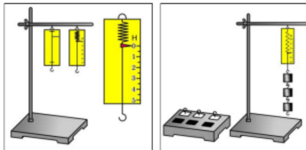
Мал. 73. Прилади до лабораторної роботи №8
