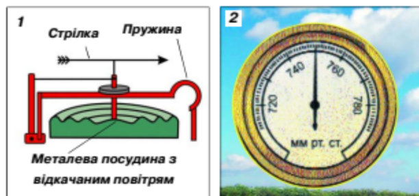
Мал. 102. Будова (1) та зовнішній вигляд (2) барометра-анероїда
