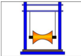
Мал. 112. Прилад для спостереження перетворень механічної енергії
