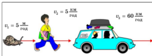
Мал. 33. Швидкість механічного руху різних тіл
