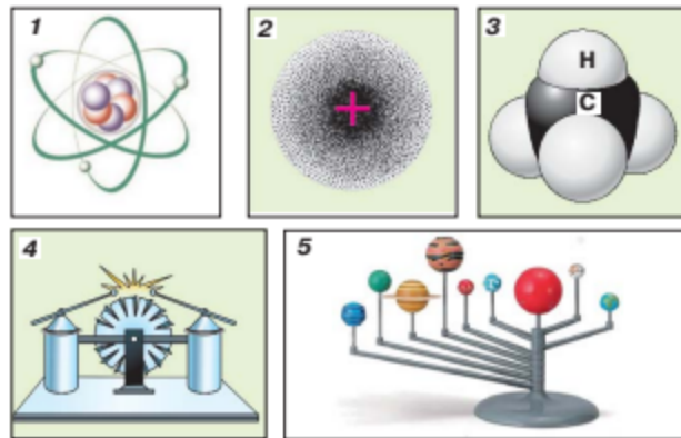
Мал. 5. Моделювання об'єктів та явищ: 1 — атома Літію (планетарна, запропонована Резерфордом); 2 — атома Гідрогену (хвильова); 3 — молекули метану; 4 — електричного розряду; 5 — Сонячної системи
