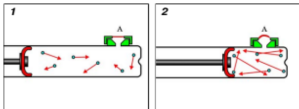
Мал. 95. Тиск газу на стінки посудини залежить від кількості молекул в одиниці об'єму
