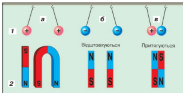
Мал. 51. 1 — взаємодія заряджених тіл (тіла заряджені: а — позитивно, б — негативно, в — позитивно і негативно); 2 — магніти та їх взаємодія
