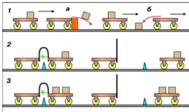
Мал. 64. Спостереження прояву явища інерції
