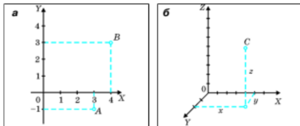
Мал. 29. Координати точки
