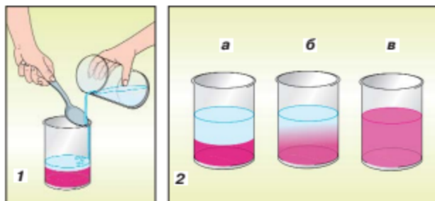
Мал. 13. Дифузія в рідинах
