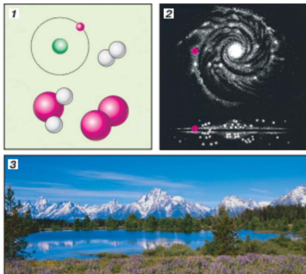
Мал. 3. 1 — атом, молекули; 2 — вигляд нашої Галактики з космічного простору (червоним обведено місцезнаходження Сонячної системи); 3 — об'єкти макросвіту
