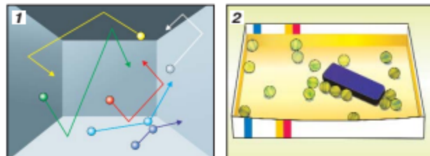
Мал. 14. Моделі броунівського руху частинок
