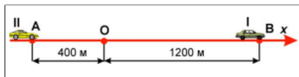
Мал. 28. До визначення положення тіла
