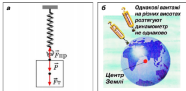
Мал. 85. Вага тіла (а), залежність ваги і сили тяжіння від висоти над поверхнею Землі (б)
