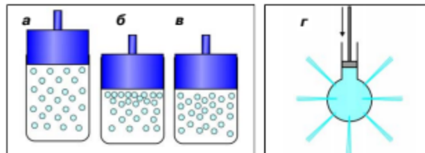
Мал. 94. Тиск газу або рідини у закритій посудині
