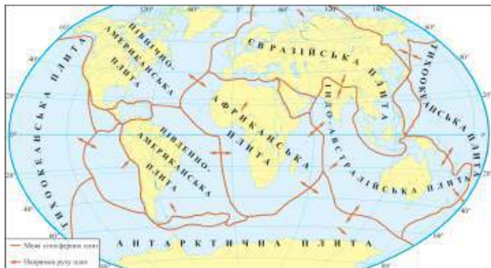
Мал. 50. Карта літосферних плит
