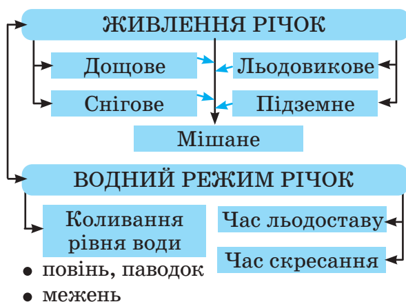
Мал. 160. Живлення та режим річок
