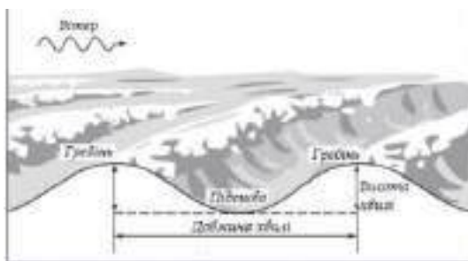
Мал. 140. Будова хвилі
