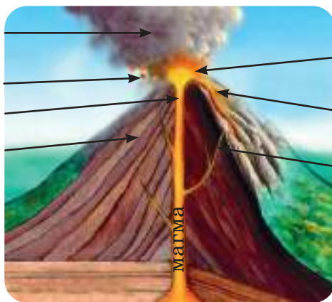
Мал. 56. Будова вулкана в розрізі
