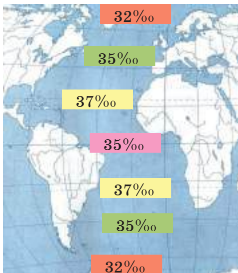
Мал. 139. Солоність водних мас Світового океану
