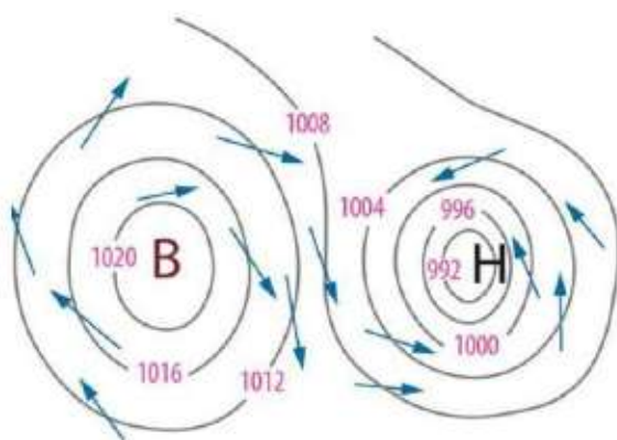
Мал. 126. Схематичне зображення ізобар, які обмежують циклони і антициклон. Сині стрілки показують напрямки вітрів, які залежать від положення областей атмосферного тиску
