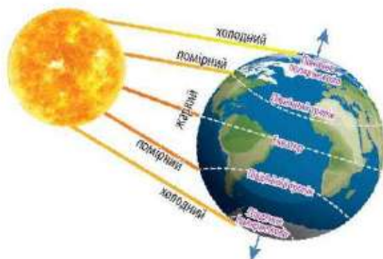
Мал. 19. Виділення поясів освітленості (теплових поясів)
