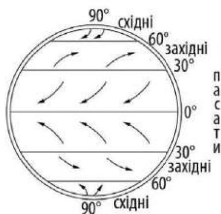
Мал. 131. Напрямки дії постійних вітрів
