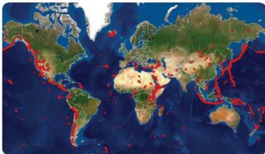
Мал. 55. Розміщення вулканів на Землі
