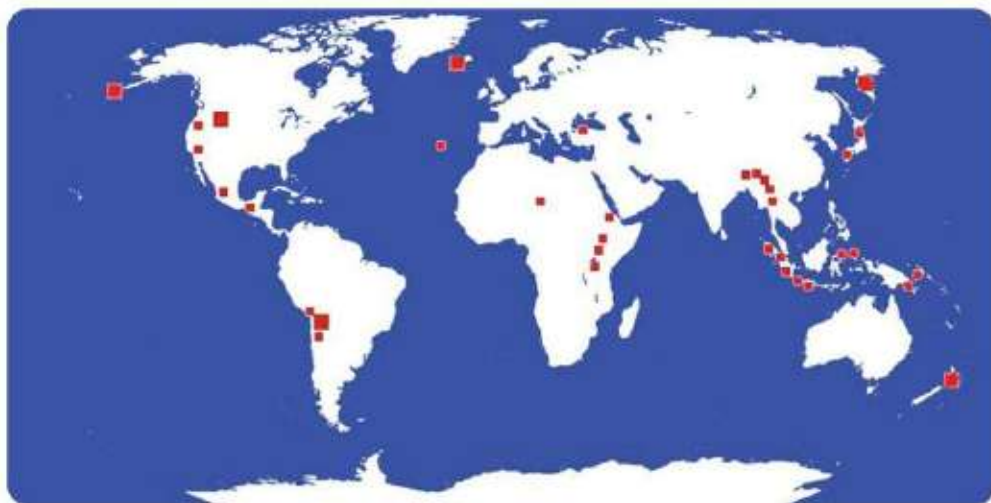
Мал. 61. Поширення гейзерів на Землі
