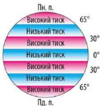
127. Смуги тиску на земній кулі
