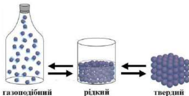
Мал. 138. Вода у трьох агрегатних станах
