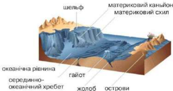
Мал. 107. Форми рельєфу океанічного дна
