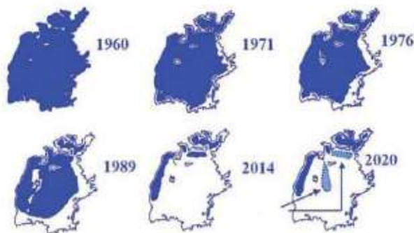
Мал. 220. Зміни розмірів Аральського моря упродовж 1960–2020 рр. На місці раніше висохлої ділянки у 2020 році, імовірно, почалося утворення ще двох мілководних водойм.
