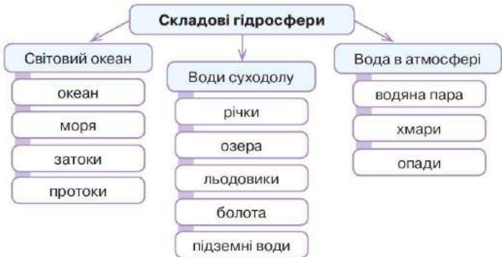
Мал. 170. Складові гідросфери
