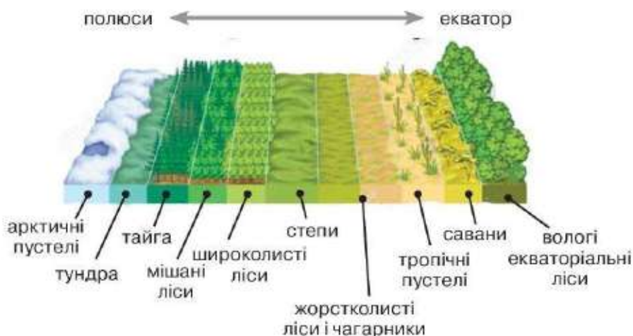
Мал. 250. Широтна зональність географічної оболонки
