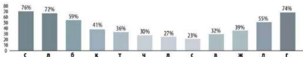
Мал. 143. Переважаюча хмарність у Полтаві упродовж року
