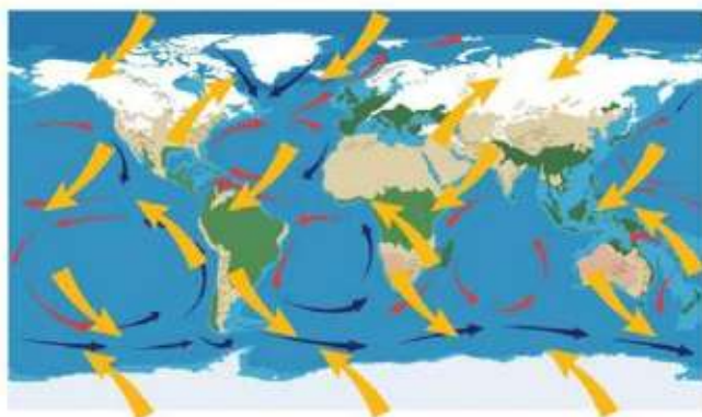
Мал. 185. Схематичне зображення напрямків постійних вітрів і найбільших океанічних течій
