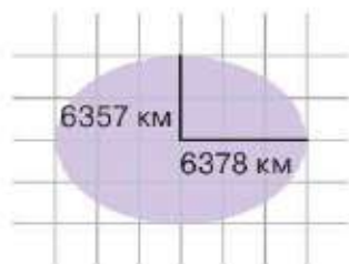
Мал. 12. Схематичне зображення еліпса з двома значеннями радіусів Землі (полярного і екваторіального)
