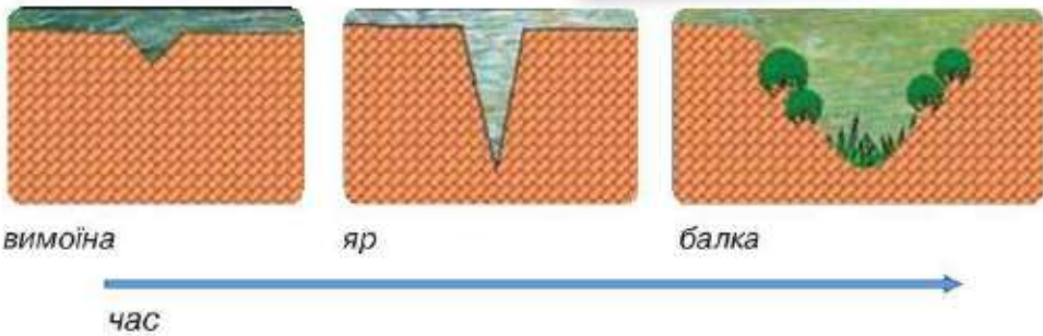
Мал. 69. Процес утворення ярів і балок
