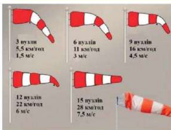
Мал. 135. Положення вітровказу за різної швидкості вітру
