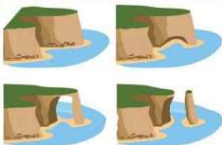
Мал. 71. Процес руйнування берегів і утворення прибережних скель
