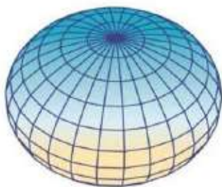
Мал. 11. Фігура еліпсоїд обертання
