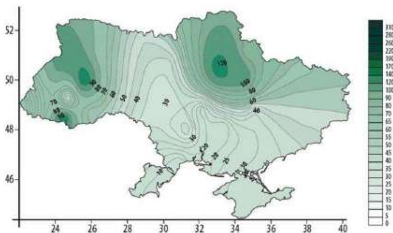
Мал. 151. Розподіл кількості опадів за липень 2022 року в Україні
