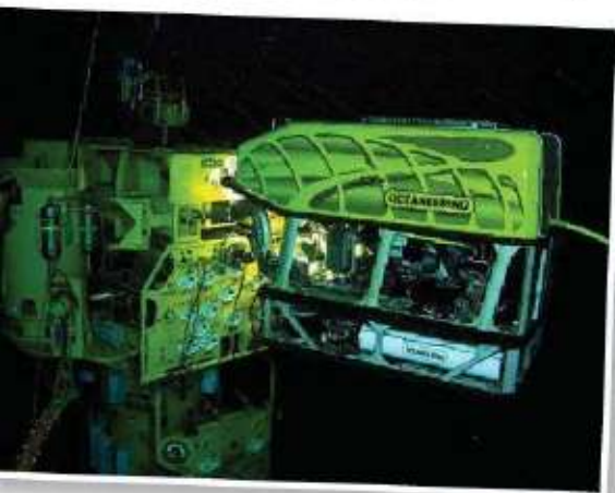
Мал. 172. Дистанційно керований підводний апарат для дослідження родовищ нафти
