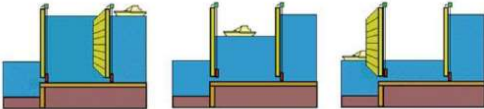
Мал. 227. Схема роботи шлюзів
