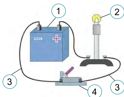
Мал. 31. Приклад електричного кола:
