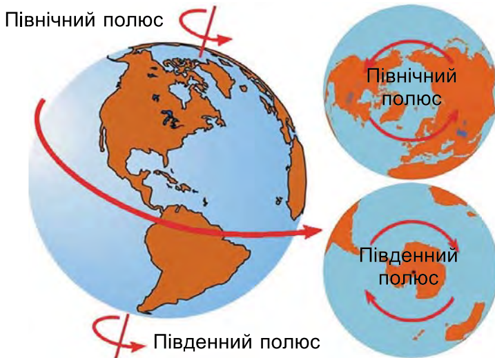
Мал. 80. Добове обертання Землі. Зверни увагу, що вісь обертання має певний кут нахилу до уявної площини, на якій міститься Земля
