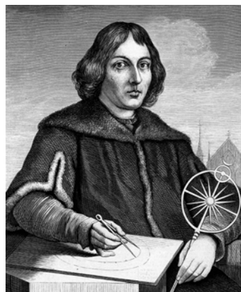
Мал. 136. А. Геліоцентрична система світу, в якій планети обертаються навколо центрального світила – Сонця, а всі зірі лежать на дуже віддаленій сфері. Б. Миколай Коперник – усесвітньо відомий астроном
