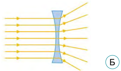
Мал. 54. А. Збиральна лінза. Б. Розсіювальна лінза
