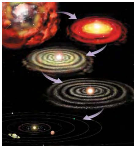
Мал. 131. Схема формування Сонячної системи
