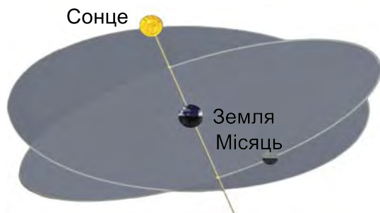
Мал. 87. Взаємне розміщення орбіт Землі та Місяця у міжпланетному просторі
