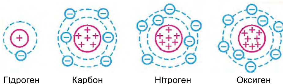
Мал. 21. Моделі атомів
