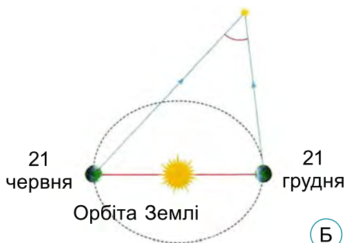
Мал. 137. Визначення відстані до недоступного об'єкта на поверхні Землі (А) та до однієї з найближчих зір (Б)
