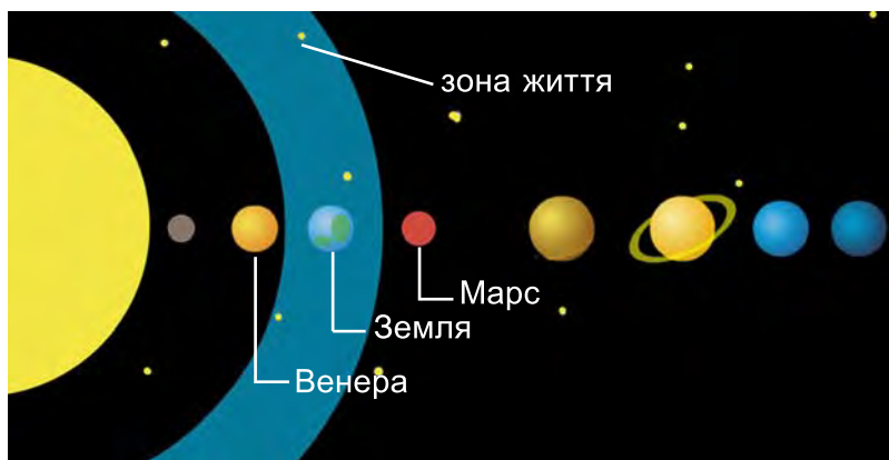
Мал. 132. Зона життя в Сонячній системі
