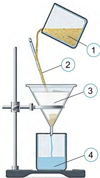
Мал. 74. Прилад для фільтрування
