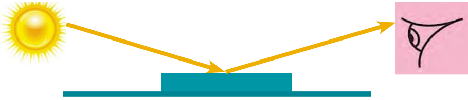
Мал. 49. Схема відбивання світла від предметів
