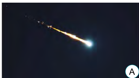
Мал. 125. А. Яскравий метеор на зоряному небі Землі. Б. Зразок метеорита
