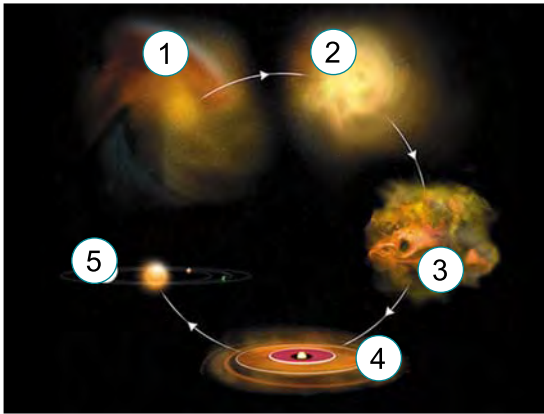
Мал. 138. Етапи формування зорі та її планетної системи.
