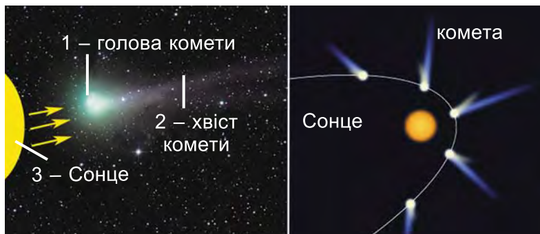
Мал. 124. Будова комети. Коли голова комети (1) рухається навколо Сонця, то її хвіст (2) спрямований у протилежний від Сонця (3) бік
