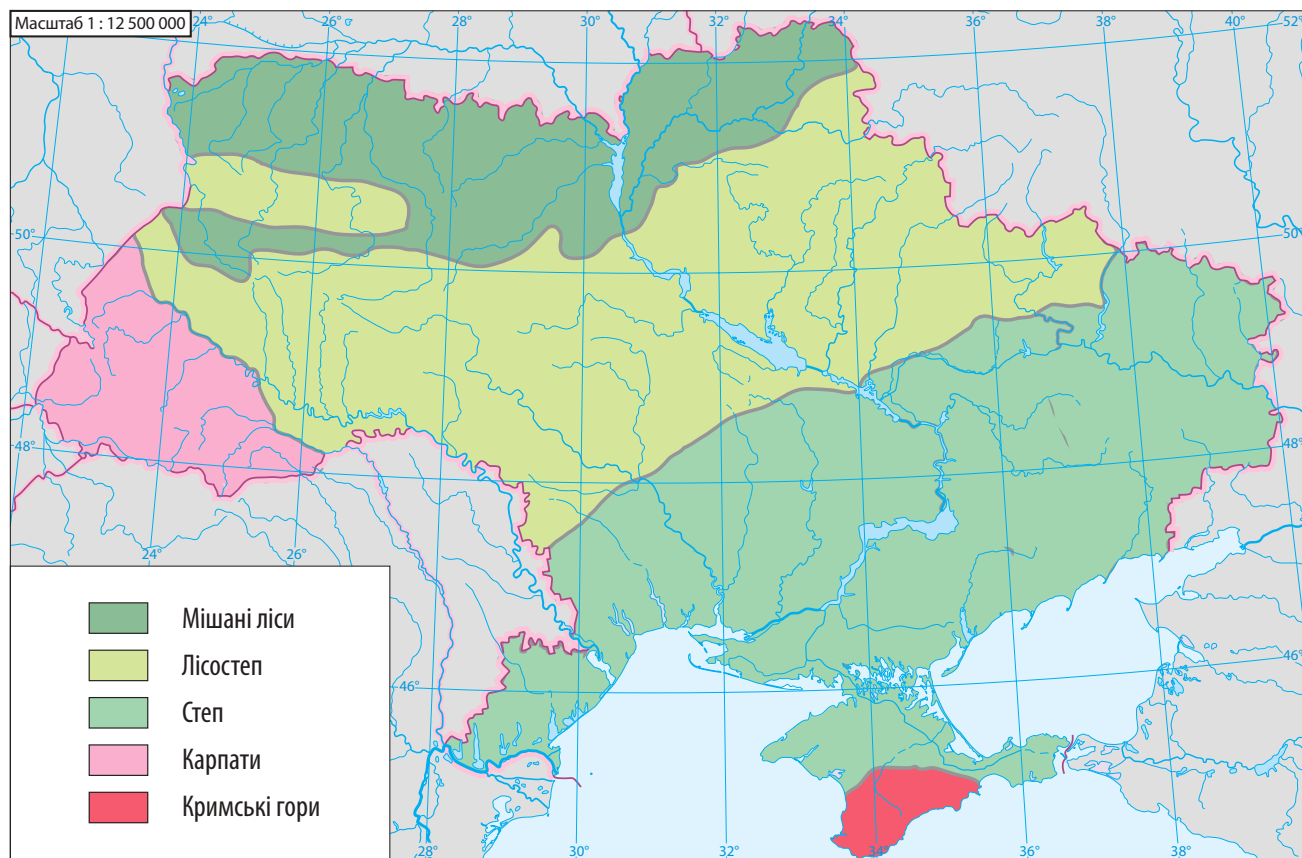
Природні зони на території України
