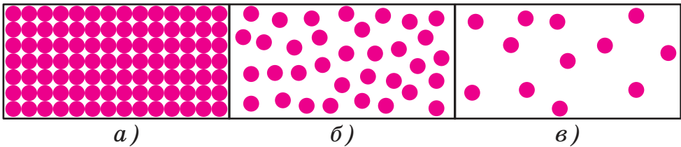
Мал. 3. Розташування частинок у твердих тілах (а), рідинах (б) і газах (в)
