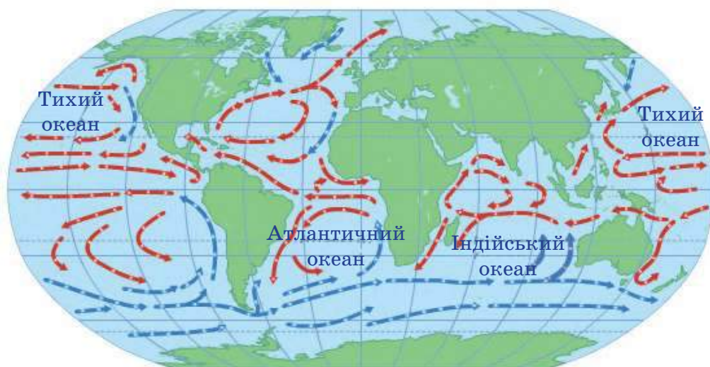
Мал. 22. Схема течій Світового океану
