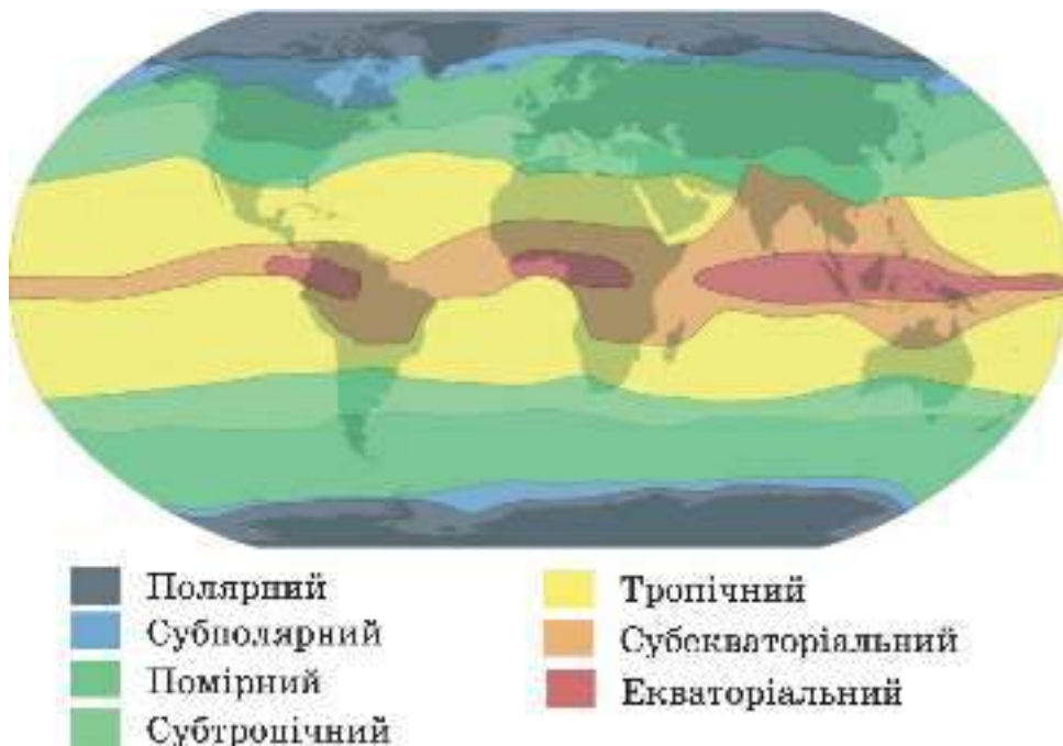
Мал. 28. Кліматичні пояси Землі
