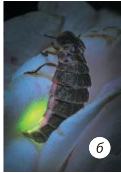
Мал. 16.1. Природні джерела світла: полярне сяйво в Норвегії (а), світлячок на квітці (б)
