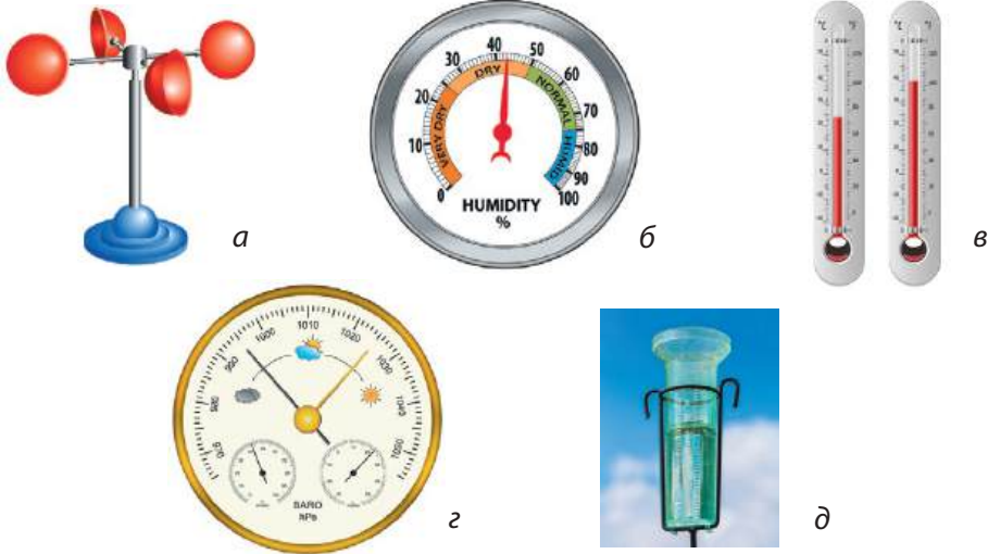
Мал. 22.2. Метеорологічні прилади: анемометр (а), барометр (б), термометри з різними рівнями вимірювання температури (в), гігрометр (г), опадомір (д)
