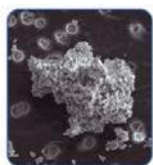
Космічний пил
