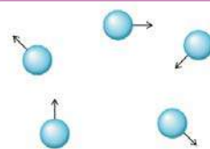
Мал. 54. Модель газу
