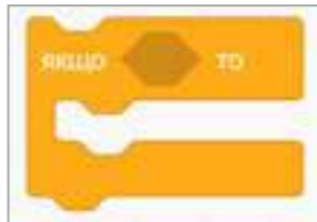
Неповне розгалуження
