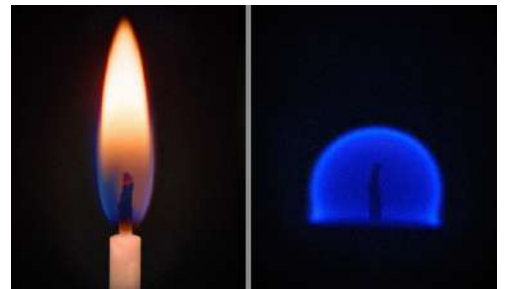
Мал. 18.2. Горіння свічки на Землі (ліворуч) та в умовах невагомості на МКС (праворуч)
