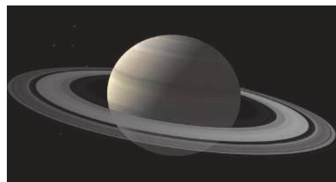
Мал. 15.4. Планета Сатурн має дивний вигляд. У Сатурну (а також в Урану) є так звані кільця. Вони складаються з величезної кількості невеликих крижинок розміром від 1 см до 10 м
