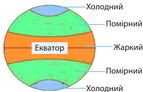
Мал. 43.2. Теплові пояси Землі
