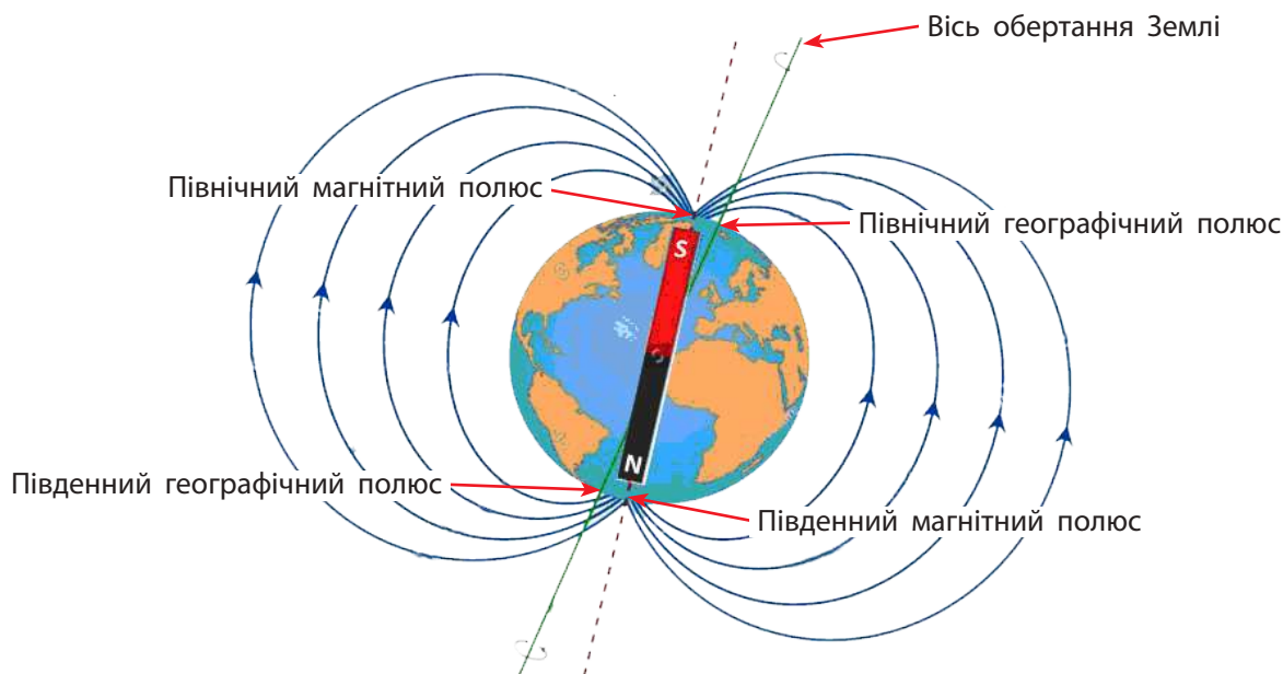
Мал. 23.5. Магнітне поле Землі
