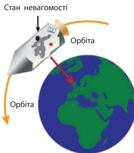
Мал. 16.4. Космічний корабель разом з екіпажем і обладнанням перебуває у стані невагомості
