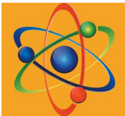
Мал. 2.1. Умовне зображення атома: усередині атома є позитивно заряджене ядро, навколо якого обертаються негативно заряджені електрони
