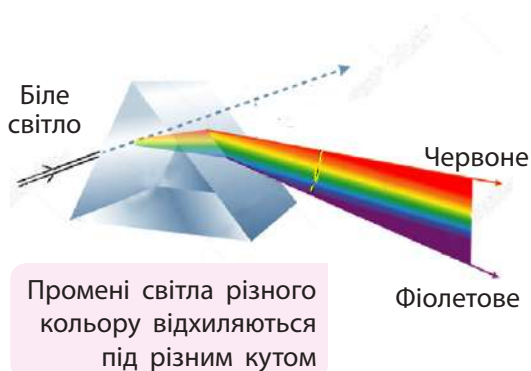
Мал. 14.1. Розділення білого світла на різні промені під час проходження крізь призму
