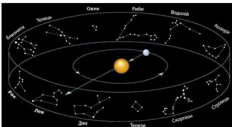
Мал. 27.4. Сонце на тлі зодіакальних сузір'їв
