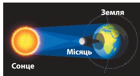
Мал. 21.4. Розташування Сонця, Місяця та Землі під час сонячного затемнення
