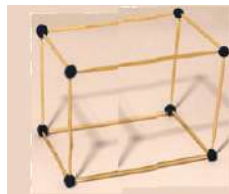
Прямокутний паралелепіпед
