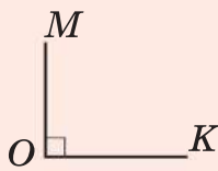
Прямий кут
