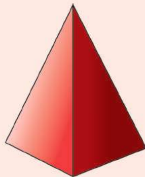
Піраміда
