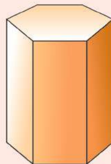
Призма
