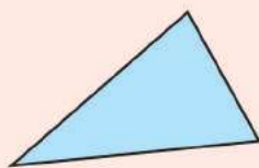
Трикутник
