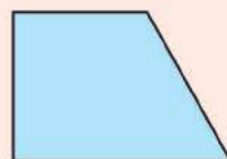
Чотирикутник
