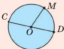
Круг
