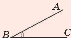
Гострий кут
