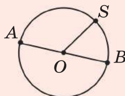
Коло
