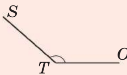
Тупий кут
