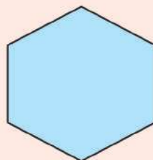
Шестикутник
