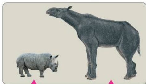
Носоріг — 2 000 кг
