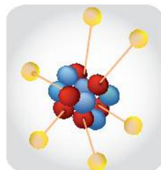
Атом вуглецю
