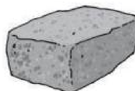
Шматок граніту
