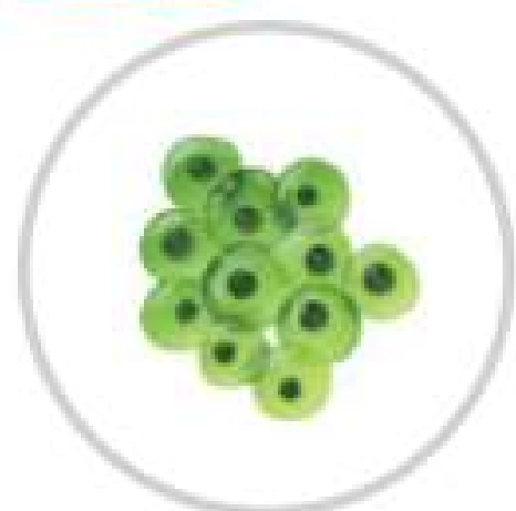
Яйця (ікра)
