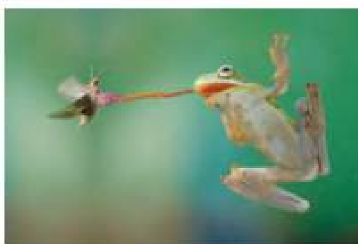
Жаба
