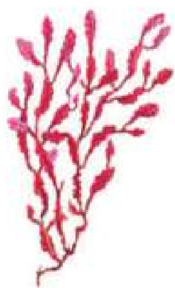
Філофора
