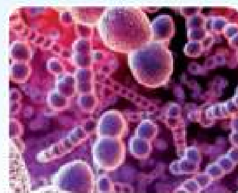
Бактерії
