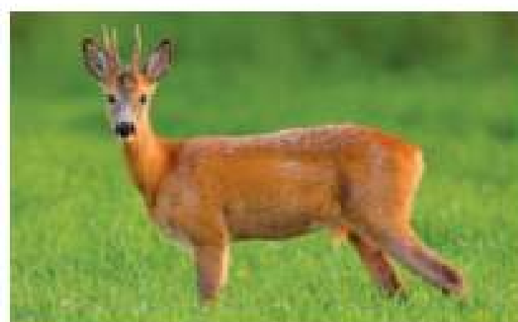
Козуля
