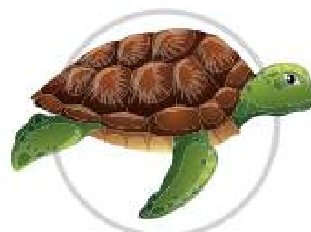
Доросла черепаха
