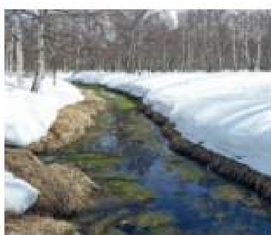
Танення снігу
