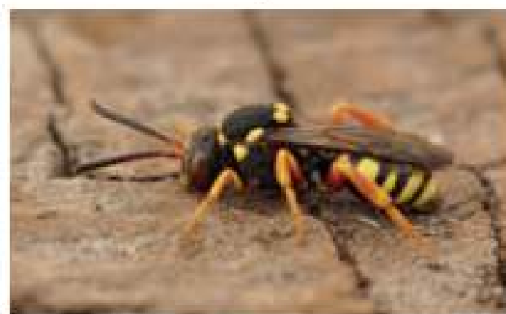
Оса
