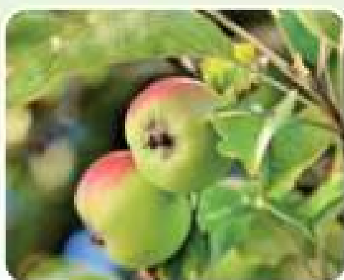
Рослини
