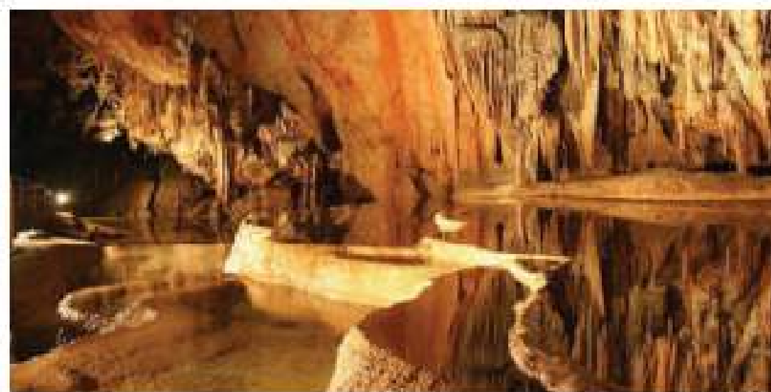
Печера
