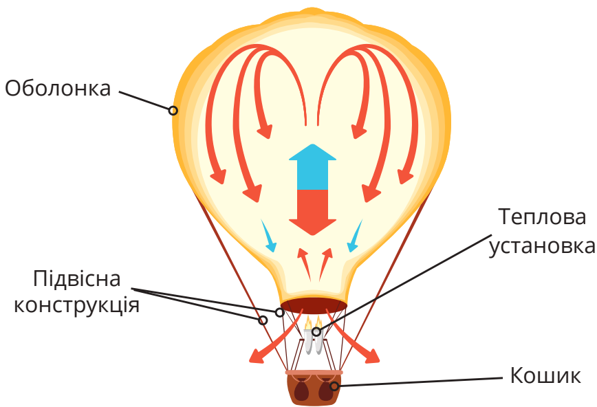
Будова аеростата
