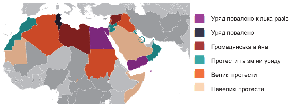
«Арабська весна» і регіональні конфлікти станом на 2014 рік, мапа Яна Ремсена
