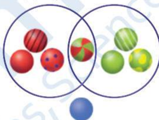
Діаграма Венна
