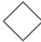
замкнена ламана
